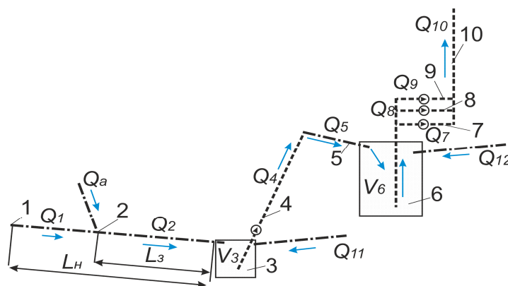
Рис. 2. Схема водоотлива из аварийной выработки: 1 – забой выработки; 2 – место прорыва воды; 3 – участковый водосборник; 4 – трубопровод участкового водоотлива; 5 – верхний насос; 6 – шахтный водосборник; 7-9 – трубы насосов шахтного водоотлива; 10 – трубопровод шахтного водоотлива; Q_1 - Q_{12} – расход воды в соответствующих ветвях сети; Q_a – аварийный поток; V_3, V_6 – вместимость водосборников, соответственно, участкового и шахтного; L_n, L_3 – протяженность подготовительной выработки и затопляемого участка
