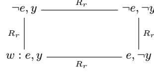
Fig. 2. Spyware example
