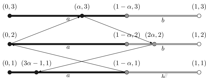
Fig. 4.4. The transformation U .
