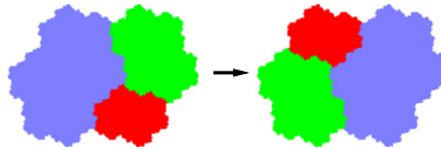
Fig. 4.3. The Rauzy fractal.
