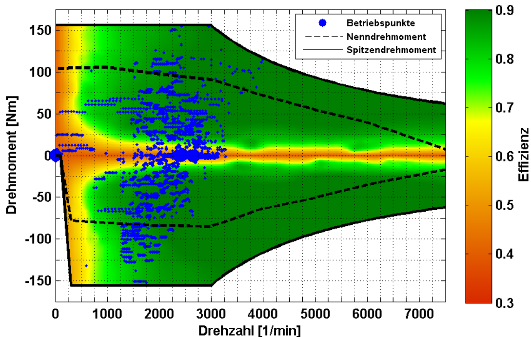
Abb. 4-85 Betriebspunkte des PHEV bei simulierter Fahrt durch den CADC-Motorway-Zyklus aufgetragen auf das Effizienzkenntfeld der elektrischen Maschine
