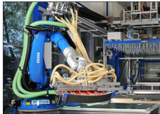
b) Draping robot
