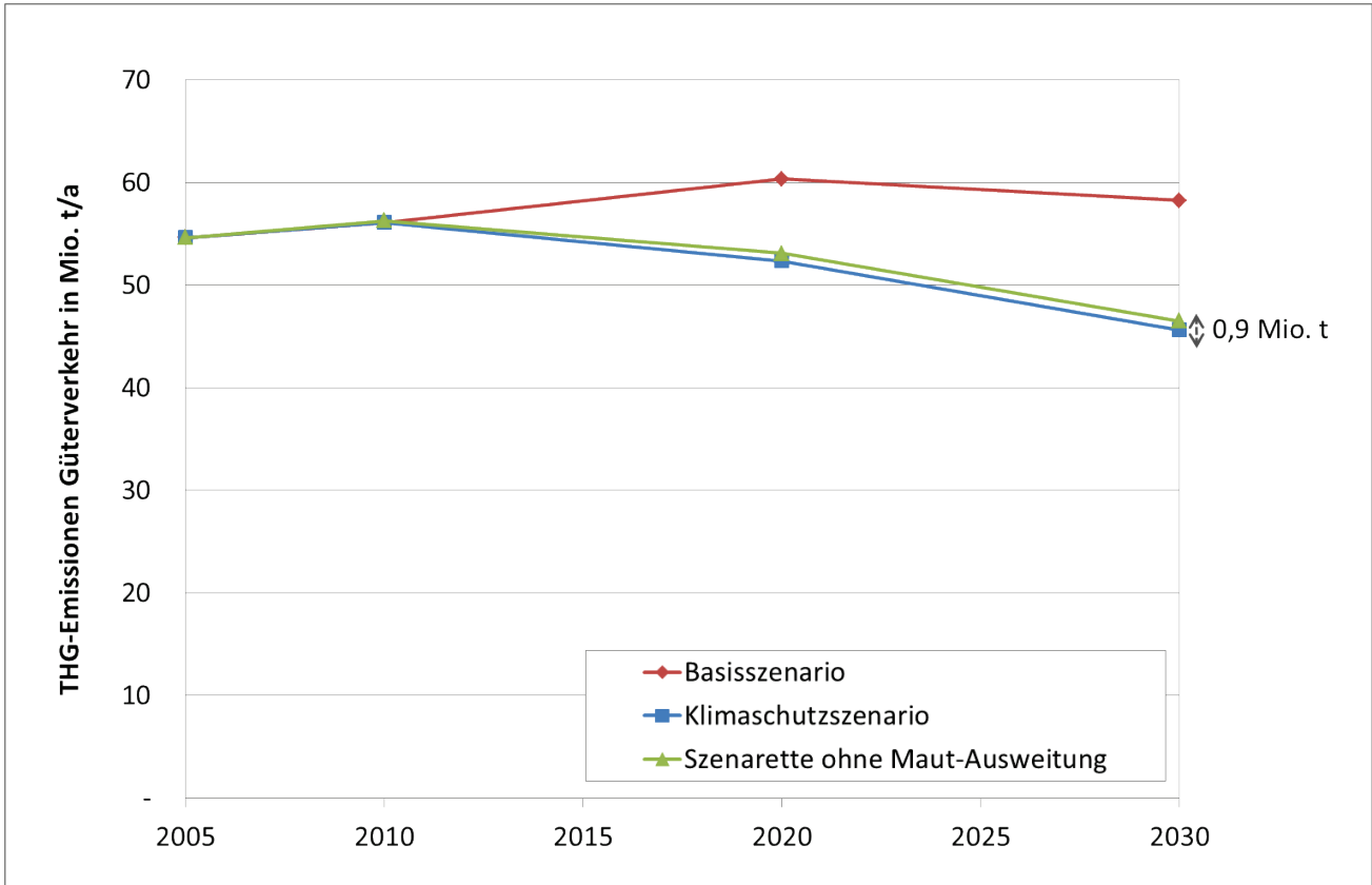
Abbildung 39: Entwicklung der Treibhausgasemissionen im Güterverkehr in der Szenarrette „auf Autobahnen beschränkte Maut“
