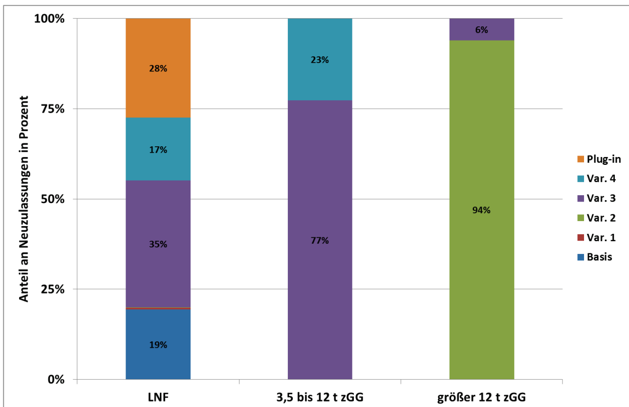
Abbildung 23: Anteile an den Fahrzeugneuzulassungen nach Effizienzvarianten im Klimaschutzszenario im Jahr 2030
