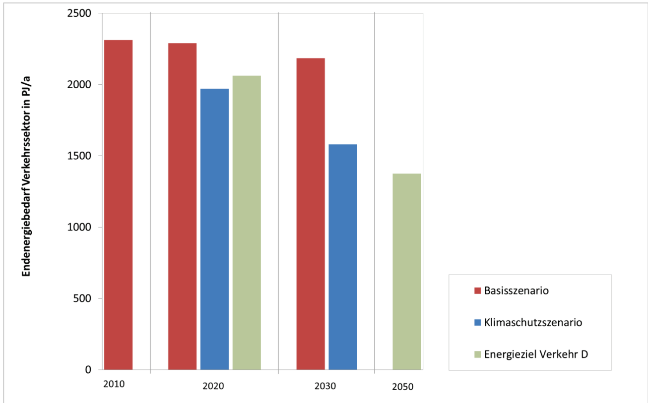
Abbildung 62: Entwicklung des Endenergiebedarfs im Basis- und Klimaschutzzenario im Kontext des Energieziels für den Verkehr
