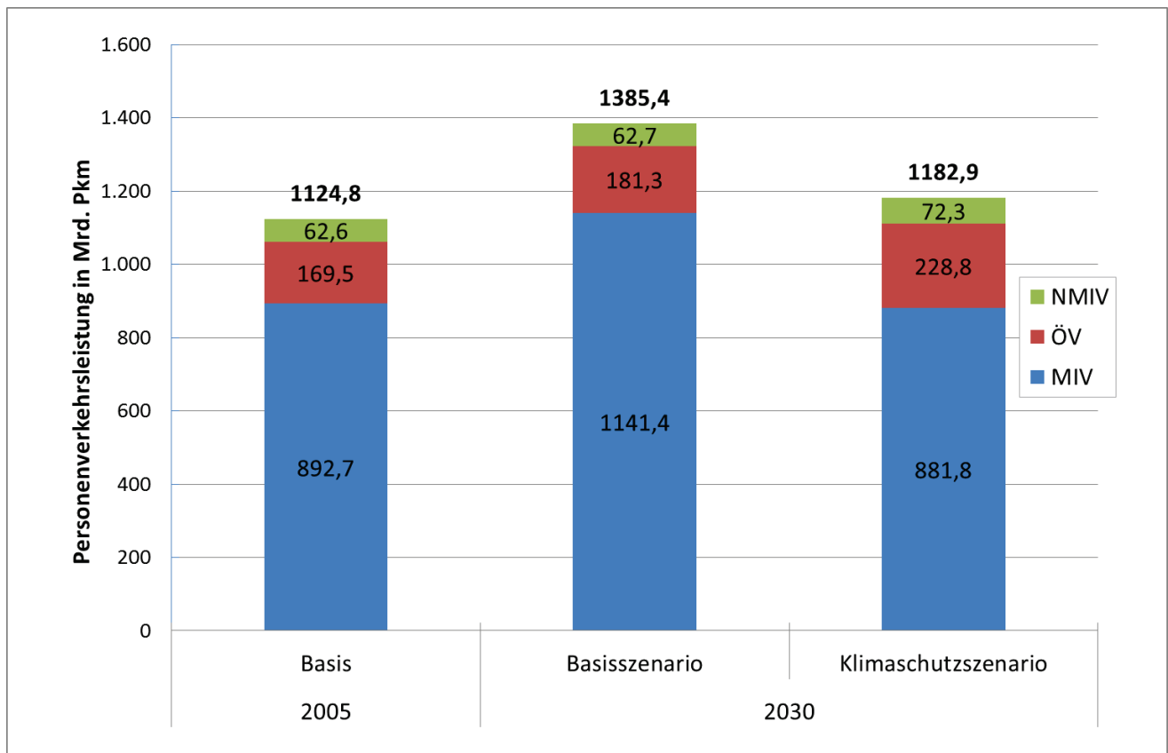
Abbildung 22: Personenverkehrsleistung im Basisszenario sowie im Klimaschutzscenario
