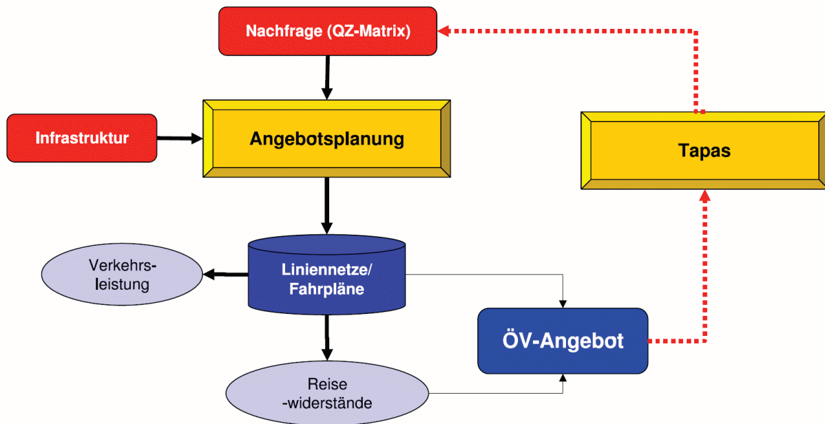
Abbildung 16: Zusammenwirken von Angebotsplanung (LINOP) und TAPAS
