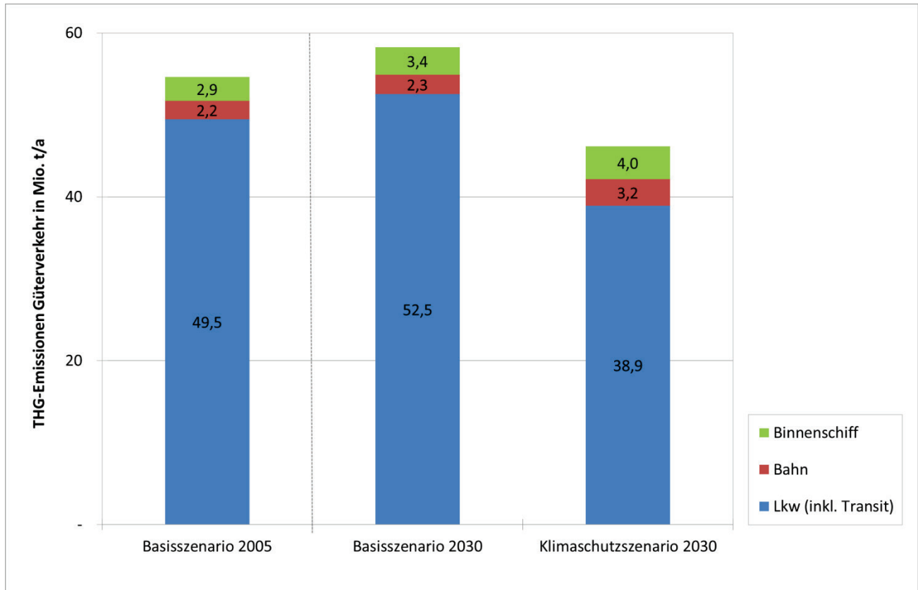
Abbildung 36: Entwicklung der Treibhausgasemissionen im Güterverkehr, differenziert nach Verkehrsmittel und Antriebstyp
