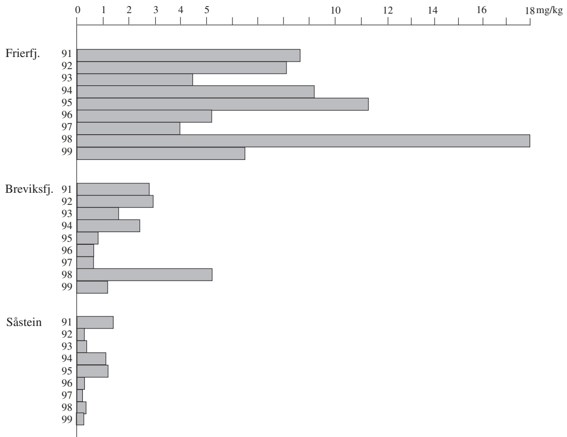
Figur 15. DCB i blandprøver av torskelerver fra Grenlandsfjordene/Telemarkskysten 1991-1999, mg/kg fett .
