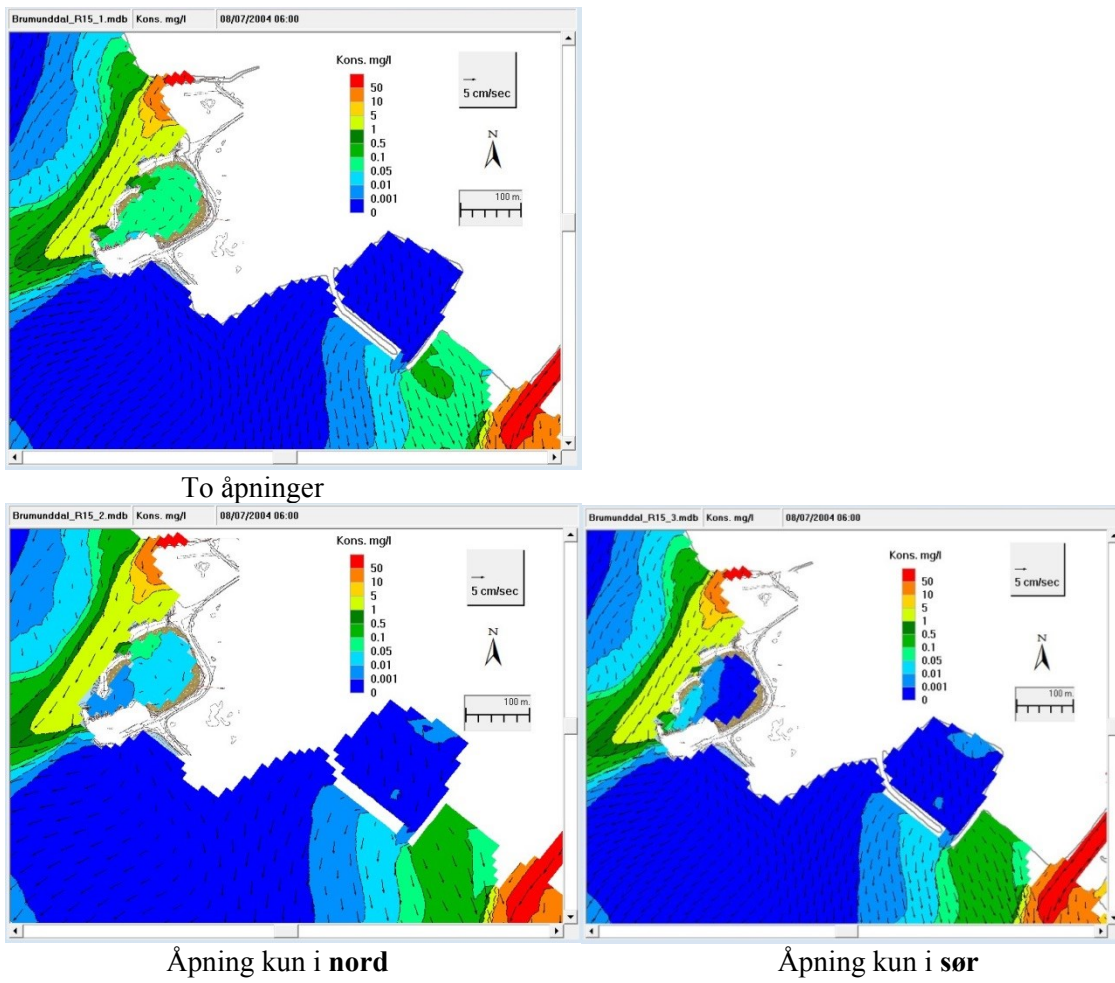
Figur 34. Bystranda ble noe påvirket av vann fra Båhusbekken ved sørgående strømmer. Påvirkningen ble redusert ved kun å ha en åpning. Ved kun åpning i sør ble påvirkningen minst.
