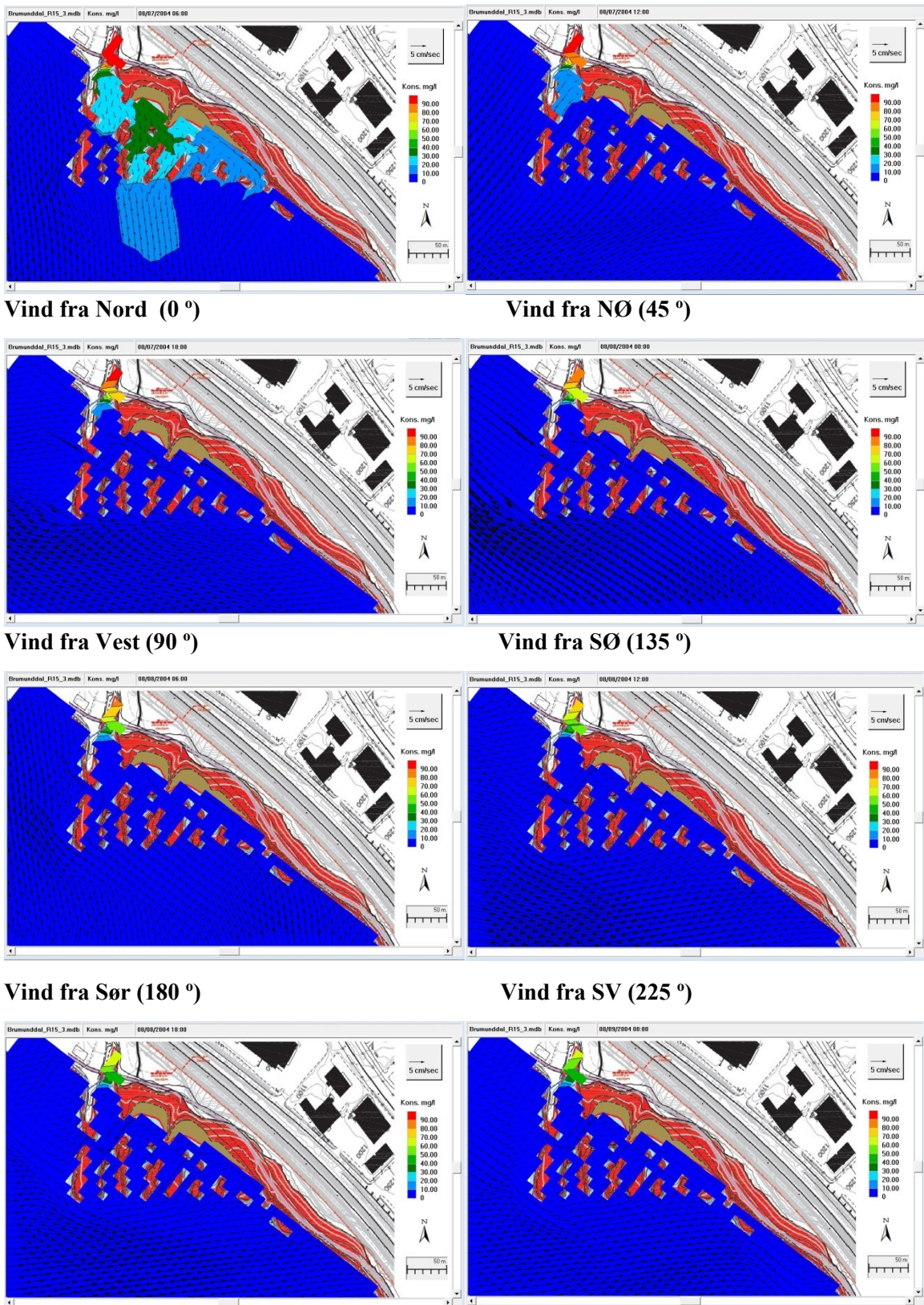
Figur 17. Holmene ved åpning i tangen i nord. Det ble små forskjeller i forhold til scenariet uten åpning i tangen.
