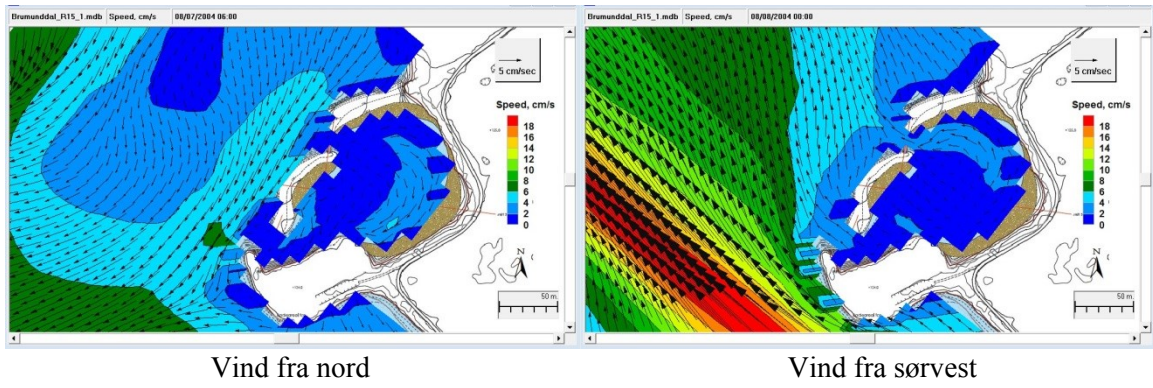
Figur 20. Vind 10 m/s. Strøm og fargeskalert fart i overflaten. Farten inne i bukta var under 4 cm/s.
