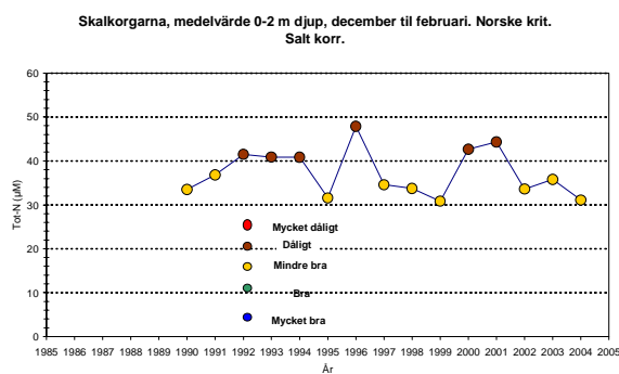
Figur 28. Mätvärden för totalkväve och nitrit plus nitratkväve ( NO_x -N) i ytvattnet (0-2 m) vid Skalkorgarna 1986/90-2004 ( \mu\text{M} ) jämförda med norska kriterier för miljöklassning (Molvær m fl 1997). Värdeklasserna är korrigerade för salthalten. Vintervärden, dec-febr.
