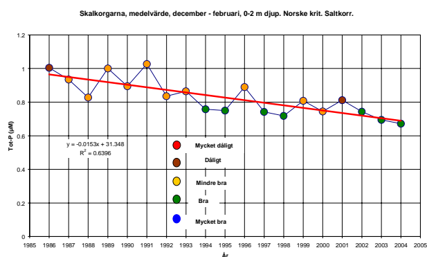
Figur 27. Mätvärden för tot-P och PO_4 -P i ytvattnet (0-2 m) vid Skalkorgarna 1986/88-2004 ( \mu\text{M} ) jämförda med norska kriterier för miljöklassning (Molvær m fl 1997). Värderingarna är korrigerade för salthalten. Vintervärden, dec-febr.
