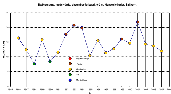
Figur 28. Mätvärden för totalkväve och nitrit plus nitratkväve ( NO_x -N) i ytvattnet (0-2 m) vid Skalkorgarna 1986/90-2004 ( \mu\text{M} ) jämförda med norska kriterier för miljöklassning (Molvær m fl 1997). Värdeklasserna är korrigerade för salthalten. Vintervärden, dec-febr.
