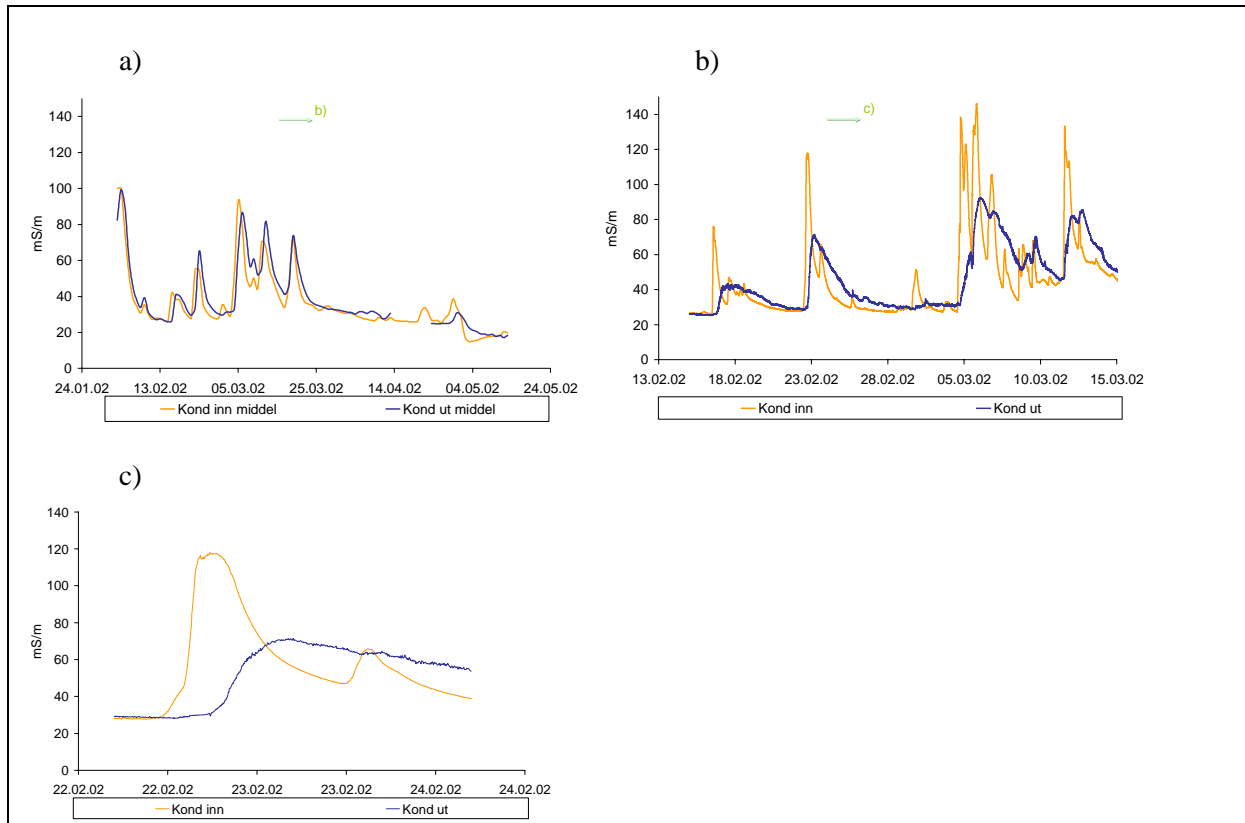
Figur 35. Data fra februar – mars 2002 med ulik grad av oppløsning: a) døgnmiddel, b) 5 – minutters intervall over ca 1 mnd., c) 5 - minuttintervall over ca 2 døgn. Farget felt angir utsnitt for neste figur.
