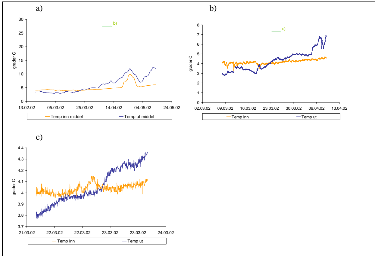
Figur 27. Data fra februar – mars 2002 med ulik grad av oppløsning: a) døgnmiddel, b) 5 - minutters intervall over ca 1 mnd., c) 5 - minuttsintervall over ca 2 døgn. Farget felt angir utsnitt for neste figur.
