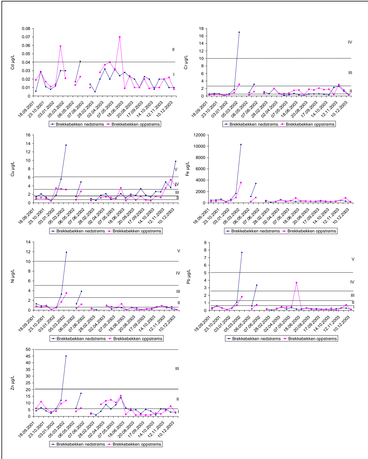
Figur 11. Konsentrasjoner av utvalgte tungmetaller 2001-2003 i Brekkebekken oppstrøms og nedstrøms E18. Vegen åpnet 31.10.2001.
