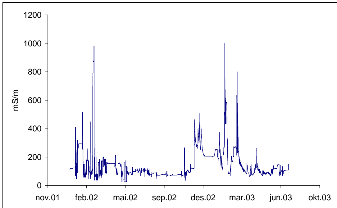
Figur 10. Konduktivitet målt ved Gutu/Skoget målestasjon i 2002 og halve 2003.
