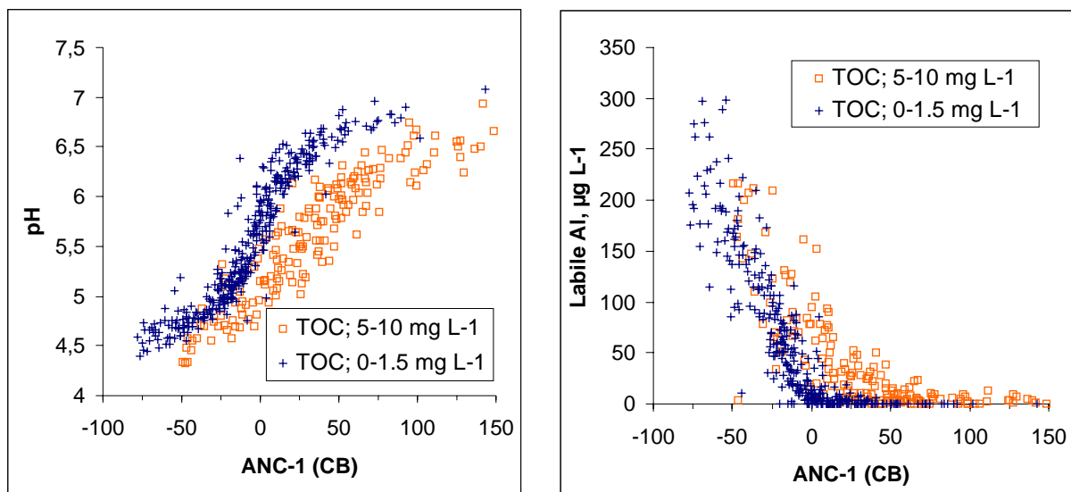
Figur 18. Sammenhenger mellom ANC og pH (a) og labilt aluminium (b) i innsjøer med en humus konsentrasjon som varierte mellom 0 og 1,5 mg C L -1 og mellom 5,0 og 10 mg C L -1 (basert på 1000-sjøers undersøkelsen i 1986).
