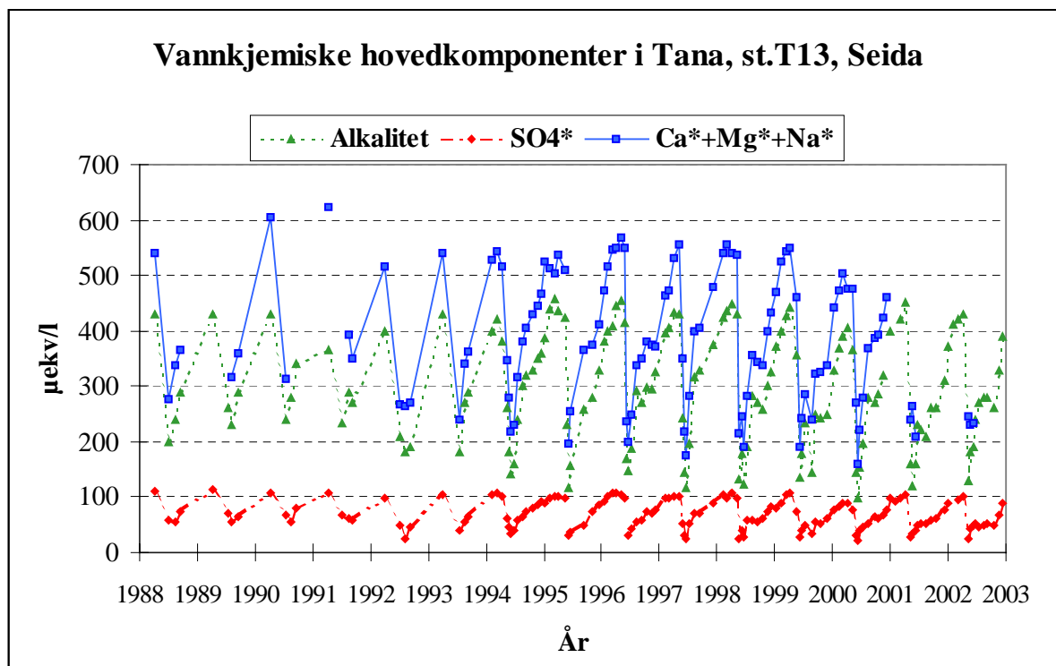
Figur 2. Vannkjemiske hovedkomponenter i Tana ved Seida (T13) for perioden 1988-2002. \text{Ca}^* + \text{Mg}^* + \text{Na}^* (sjøsaltkorrigert), \text{SO}_4^* (sulfat, sjøsaltkorrigert) og alkalitet.
