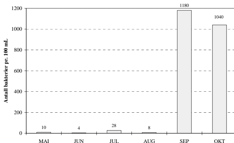
Figur 58. Termotabile kolibakterier i Iglevatn 1997 (antall bakterier pr. 100 ml).
