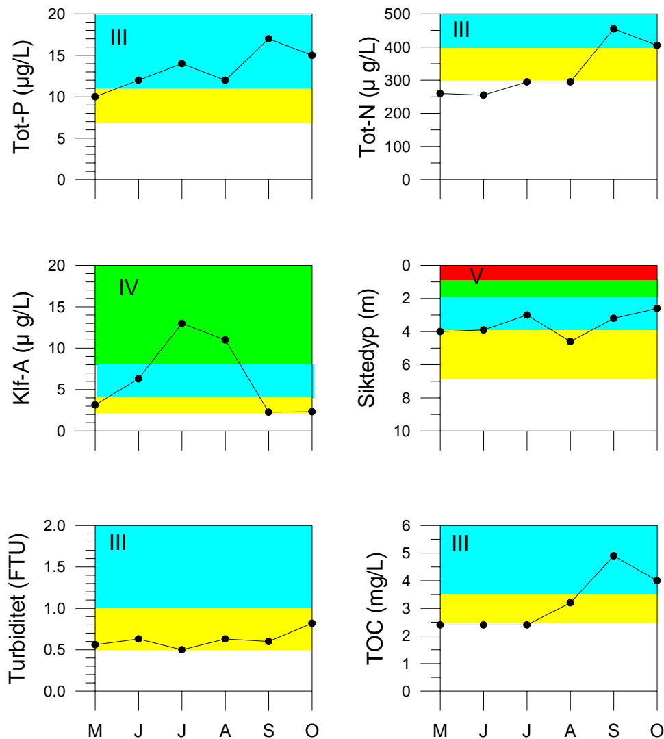
Figur 37. Vannkjemiske målinger fra Byrkjelandsvatn 1997. Øverst næringsstoffer Tot-P (til venstre) og Tot-N (til høyre), i midten Klf a (til venstre) og siktedyp (til høyre), nederst turbiditet (til venstre) og TOC (til høyre). Nivåene for tilstandsklasser er vist med skravering. Høyeste klasse på hver figur er angitt med romertall (I - V).
