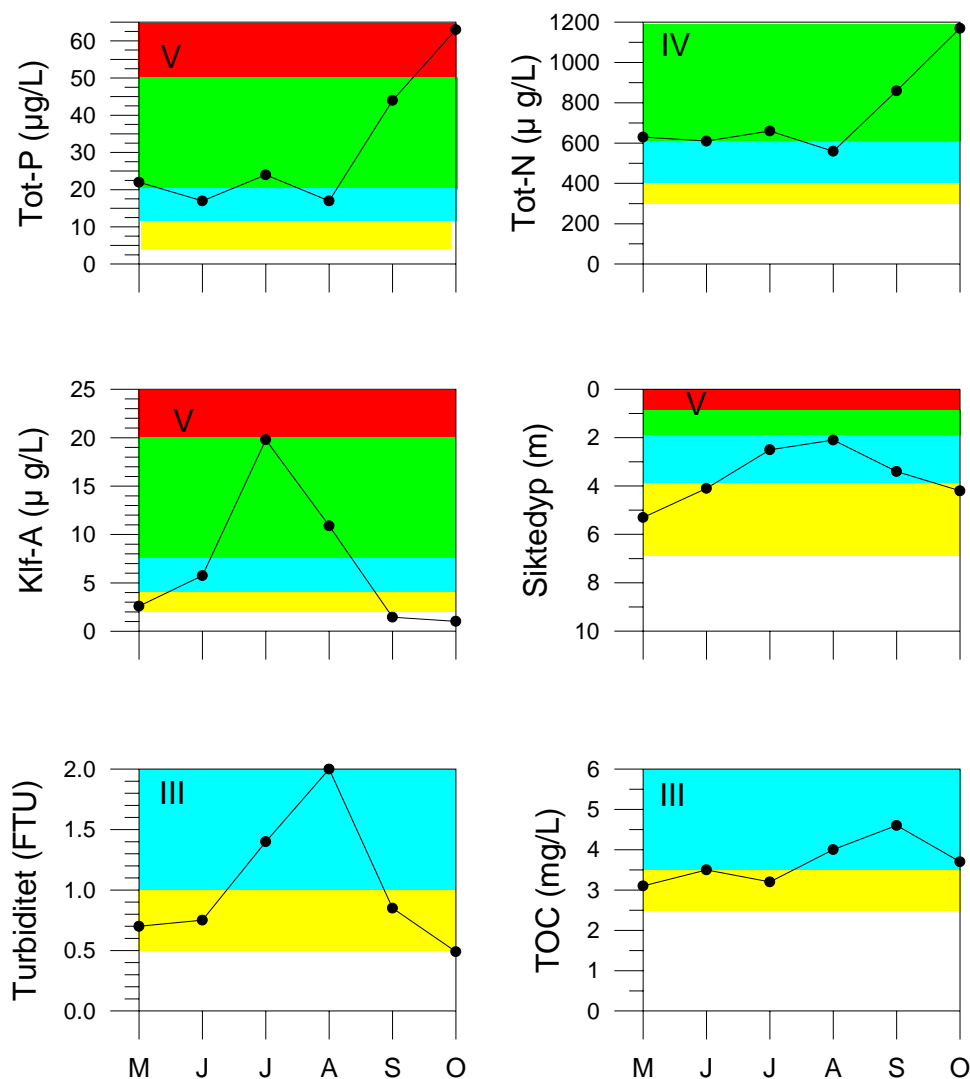
Figur 45. Vannkjemiske målinger fra Myravatn 1997. Øverst næringssaltene Tot-P (til venstre) og Tot-N (til høyre), i midten Klf a (til venstre) og siktedyp (til høyre), nederst turbiditet (til venstre) og TOC (til høyre). Nivåene for tilstandsklasser er vist med skravering. Høyeste klasse på hver figur er angitt med romertall (I - V).
