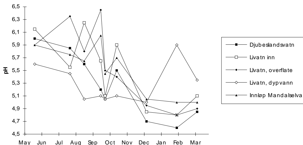
Figur 11. pH-utvikling ved forskjellige stasjoner i Høyåna i 1992-93.
