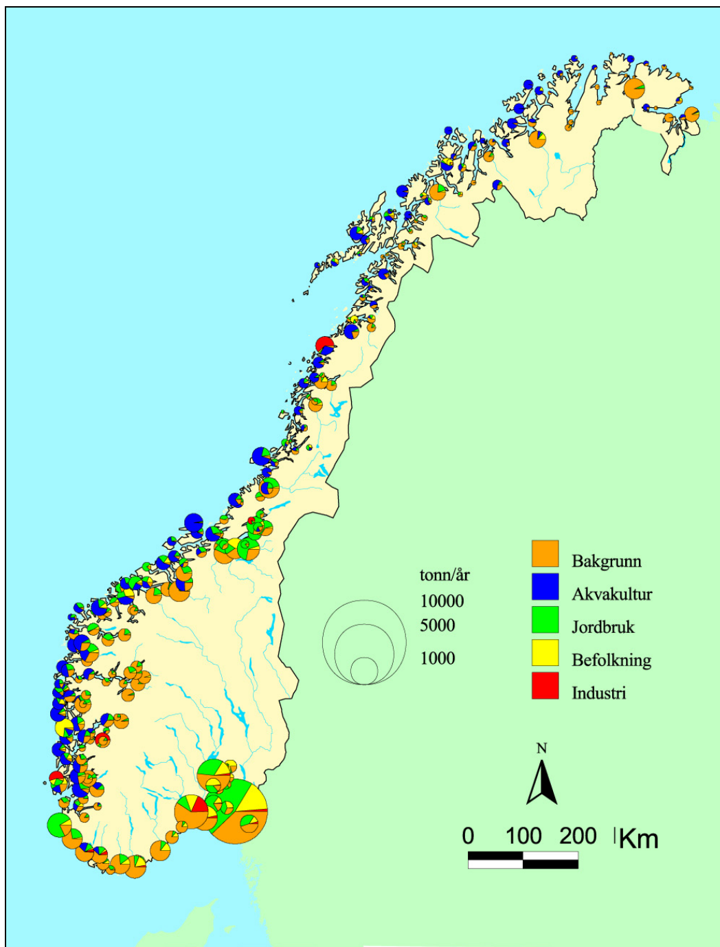
Figur 16. Den relative størrelsen av de forskjellige nitrogenkildene pr. vassdragsområde i 2002.
