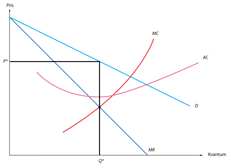
Figur 2: Monopolistens tilpasning.
