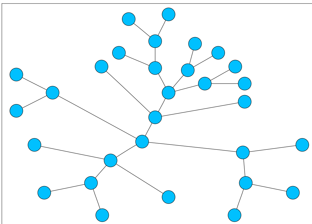
Figur 3.5: Ustrukturerte P2P-nettverk.
