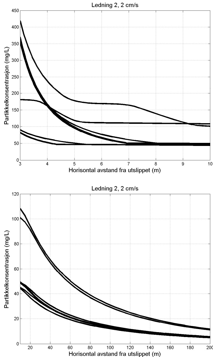
Figur 22. Beregnet partikkelkonsentrasjon ved horisontal avstand fra utslippspunktet fra oppredningsfasen i ledning 2 ved hjelp av Visual Plumes for de ulike tilfellene. Kjøringen er gjort kun for 2 cm/s med strømretningene omkring 70 og 280 grader. De ulike tilfellene er fra datoene 18.1.92, 30.11.02, 17.6.2010, 12.10.2010 og 6.12.2010. De to som grafene som skiller seg ut er fra juni med sterk sjiktning i vannsøylen. Øverst: 3-10 m fra utslippspunktet, nederst: 10-200 m fra utslippspunktet.
