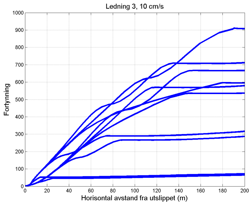
Figur 17. Fortynning av utslippet fra syrevaskfasen med strømhastighet 10 cm/s og strømrøtning 70 og 280 grader. Den sterkeste fortynningen skjer for tilfellene med grunnest innlagringsdyp. De ulike tilfellene er fra datoene 18.1.92, 30.11.02, 17.6.2010, 12.10.2010 og 6.12.2010.
