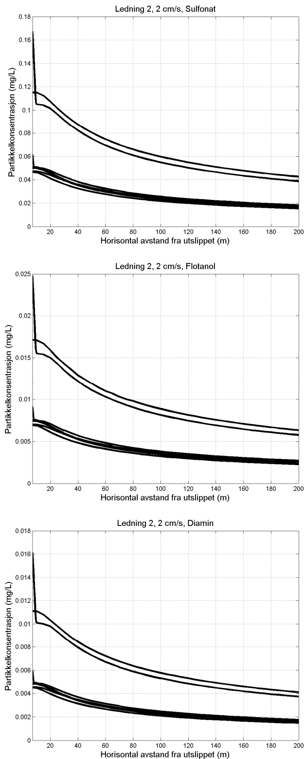
Figur 21. Fortynning av flotasjonskjemikaliekonsentrasjonene fra utslippet til oppredningsfasen i ledning 2. Øverst: sulfonat, midten: flotanol, nederst: diamin. Partikkelkonsentrasjonen er vist fra 7 til 200 meter fra utslippspunktet. Det fortynnede utslippet når opp til overflaten for noen av tilfellene. De ulike tilfellene er fra datoene 18.1.92, 30.11.02, 17.6.2010, 12.10.2010 og 6.12.2010. De to grafene som skiller seg ut for alle kjemikalierne er fra juni med svak sjiktning i vannsøylen.
