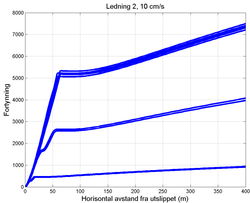
Figur 13. Fortynning av utslippet fra oppredningsfasen med strømhastighet 10 cm/s med strømretning omkring 70 og 180 grader. Fortynningen varierer for de ulike profilene vist i Figur 9 . Den sterkeste fortynningen skjer for tilfellene med grunnest innlagringsdyp. De ulike tilfellene er fra datoene 18.1.92, 30.11.02, 17.6.2010, 12.10.2010 og 6.12.2010.
