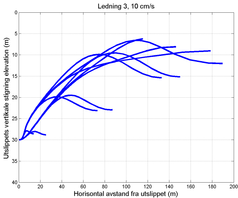
Figur 16. Innlagringsdyp av utslippet fra syrevaskfasen med strømhastighet 10 cm/s og strømretning omkring 70 og 280 grader. For dette scenarioet er det ingen av profilene som når opp til overflaten og innlagringsdypet er mellom 28 og 7 m. De ulike tilfellene er fra datoene 18.1.92, 30.11.02, 17.6.2010, 12.10.2010 og 6.12.2010.
