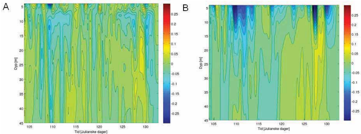
Figur 15a og b. Målt (øverste) og modellert (nederste panel) strøm fra stasjon 2 (strøm-måleren lengst nordøst) som en tidsserie med dypet. Tidsaksen viser tid i dager fra 1.1.2009 og strekker seg fra 15. april til 14. mai 2009, mens vertikalaksen begrenser dypene mellom 4 og 45 m. Strømretning er langs med fjorden med positiv retning innover mot Storfjorden, og ekvidistansen er 0.025 m/s.
