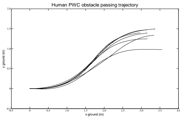
Fig. 2. Human slalom PWC trajectories
