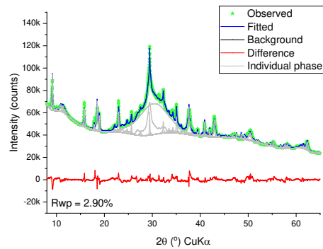
(d) 10% MgO
