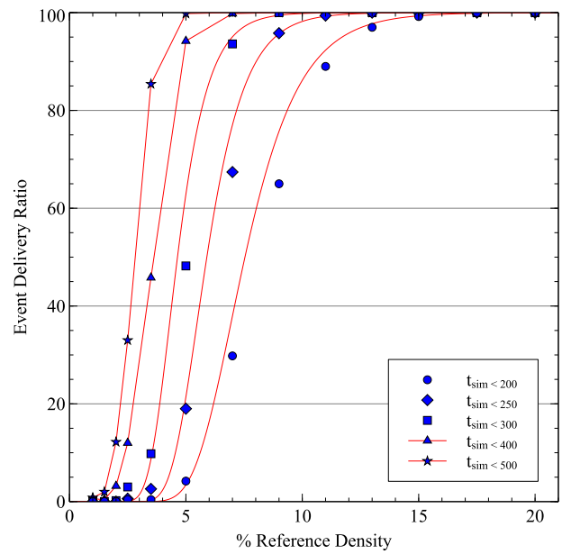
(d) Delivery Ratio of Lévy Mobility Model
