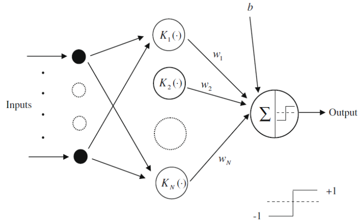
Gambar 2.7. Arsitektur SVM
