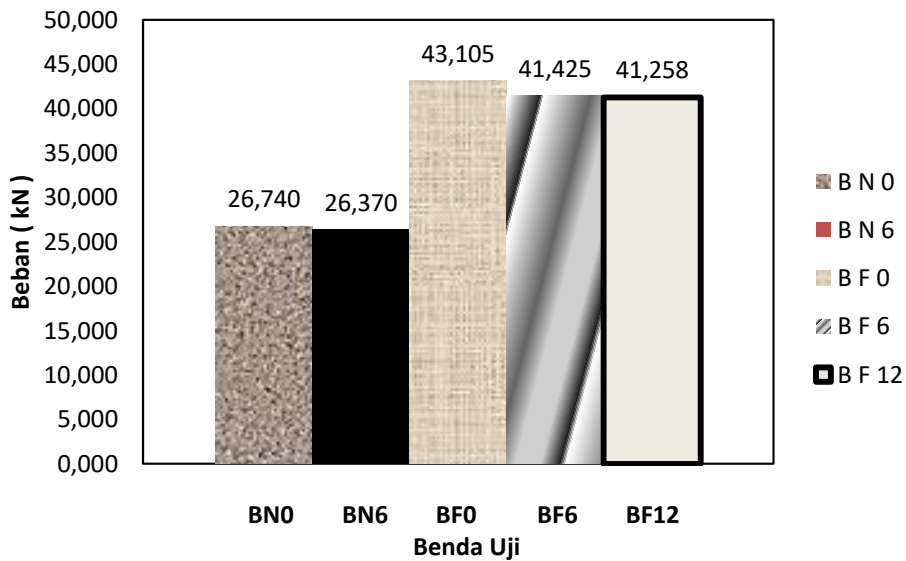
Gambar 3. Histogram Beban Maksimum
