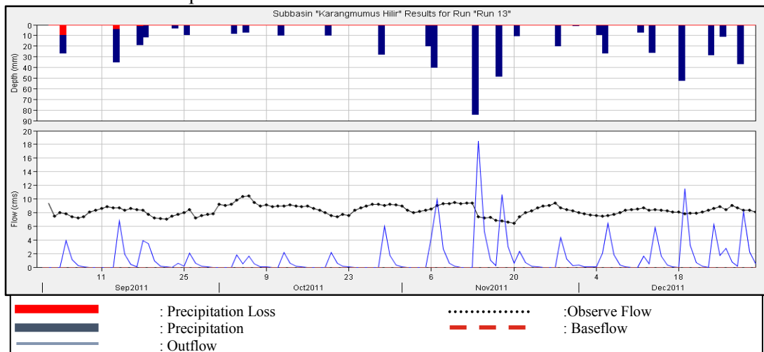
Gambar 3. Debit hasil simulasi HEC-HMS Sub-DAS Karangmumus pada Subbasin Karangmumus Hilir
