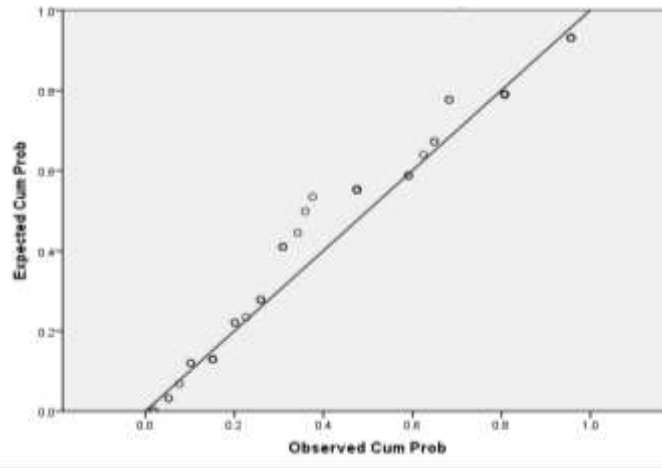
Gambar 3. Normal P-P Plot of Motivasi Belajar Belajar Siswa
