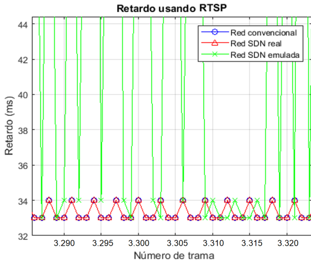
Figura 13. Acercamiento gráfico al retardo usando RTSP
