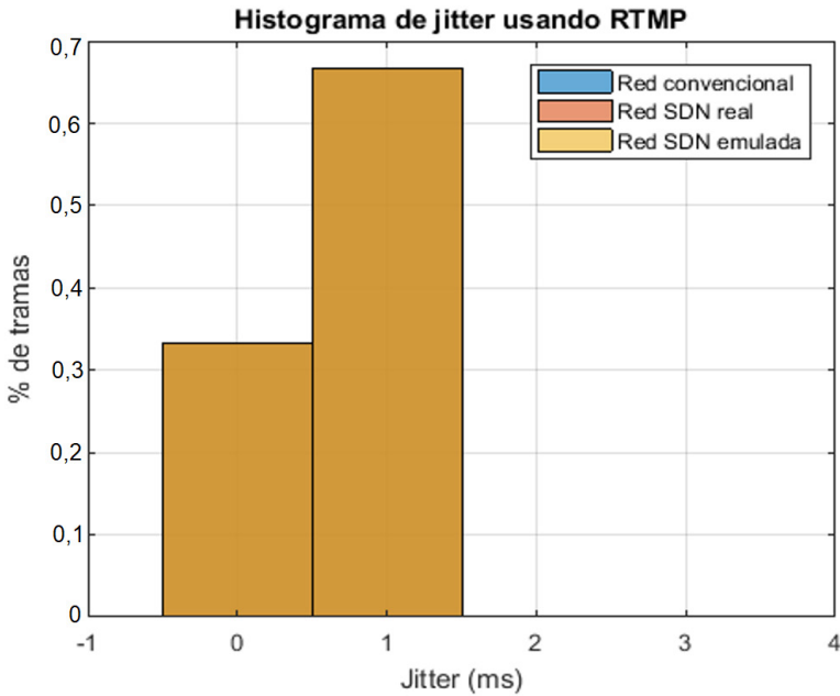
Figura 14. Histograma de jitter RTMP medido en cada escenario
