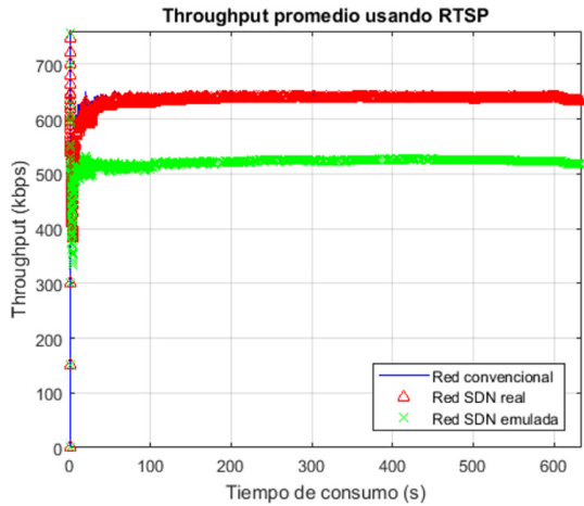
Figura 17. Rendimiento promedio usando RTSP
