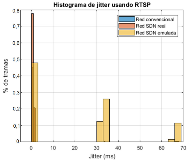
Figura 15. Histograma de jitter RTSP medido en cada escenario
