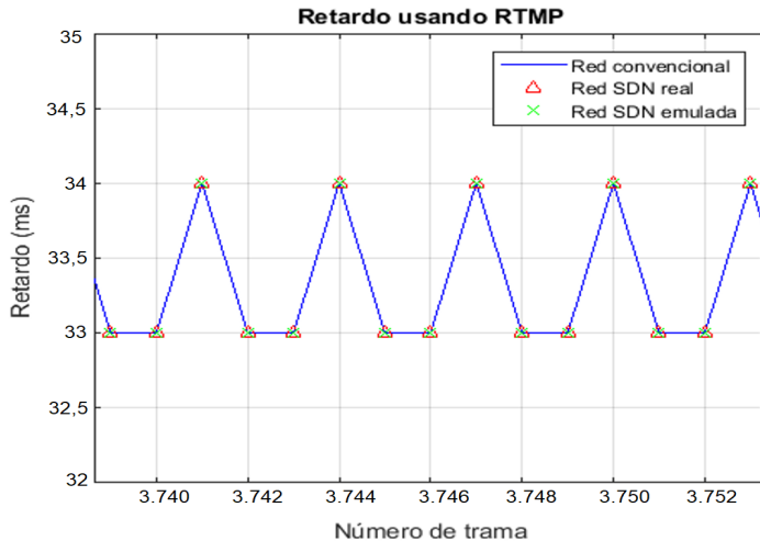
Figura 11. Acercamiento al retardo usando RTMP
