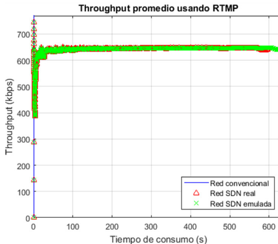
Figura 16. Rendimiento promedio usando RTMP
