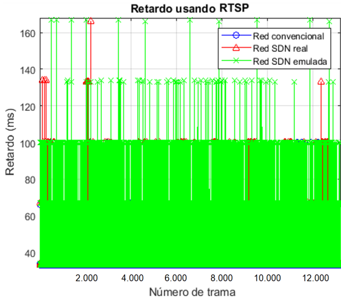
Figura 12. Retardo en escenarios con RTSP
