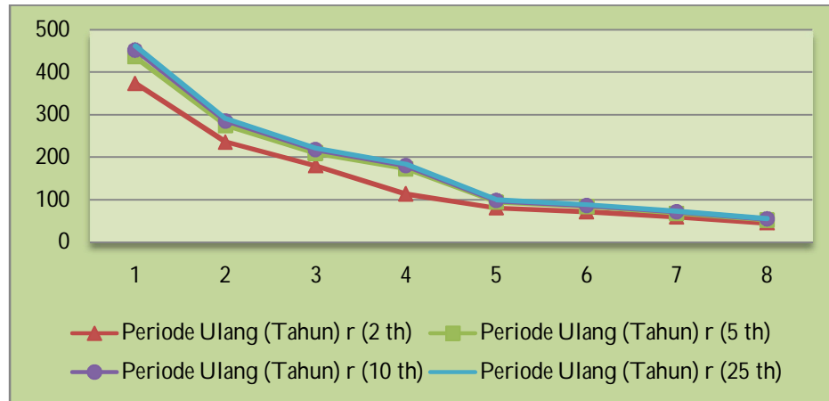
Gambar 2. Kurva IDF daerah perencanaan
