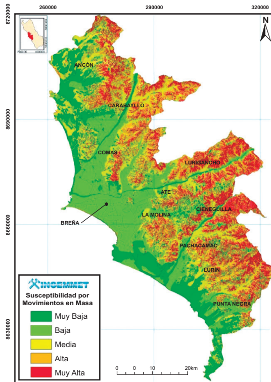
Figura N° 3. Mapa de susceptibilidad a los movimientos en masa de Lima Metropolitana y el Callao (Villacorta et al., 2014). En rojo: las zonas de arranque más susceptibles por movimientos en masa. En amarillo: sectores sensibles a los depósitos de los huaycos detonados por lluvias excepcionales (ENSO).
