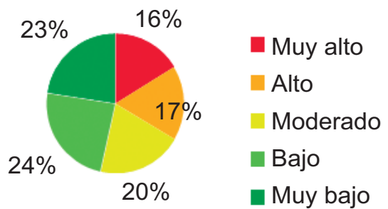
Figuras N° 4 y N° 5. Superficie total y frecuencia de movimientos en masa en los cinco niveles de susceptibilidad.
