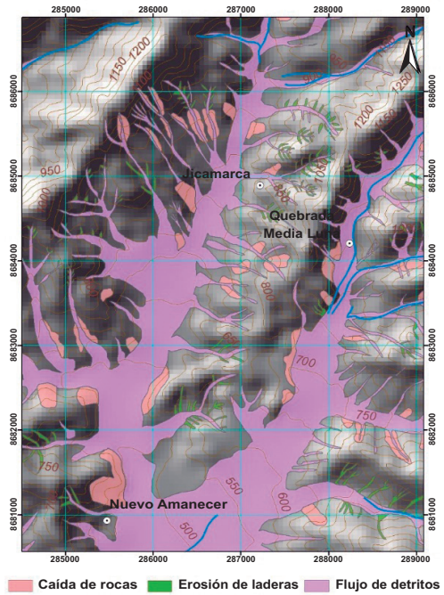
Figura N° 1. Flujos de detritos, caídas de rocas por gravedad y cárcavas, identificadas en imágenes satelitales y confirmadas por trabajos de campo en las quebradas Jicamarca y Media Luna (San Juan de Lurigancho).
