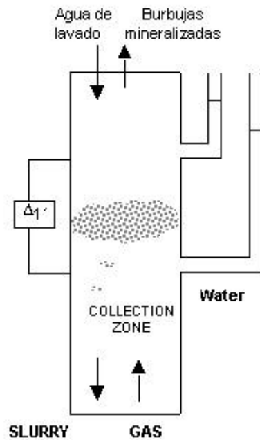
Figura N.º 3. Medida de la presión del gas y dirección de flujo en celda-columna (22)
