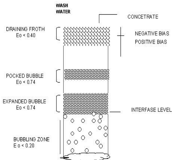
Figura N.º 4. Perfil de la zona de la espuma y anatos 1985 (6)
