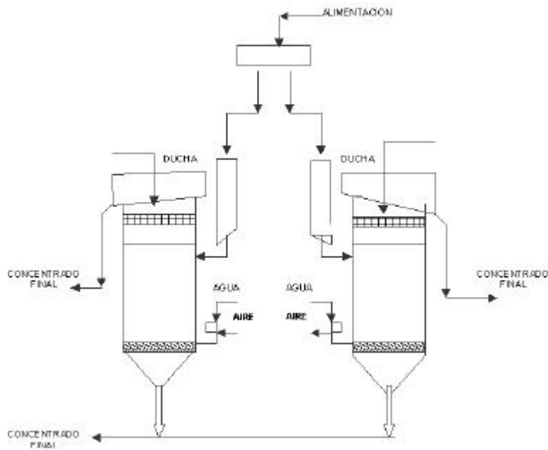
Figura N.º 7 Instalación en paralelo (18)
