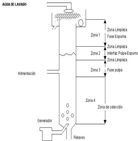
Figura N.º 2. Zonas de la celda-columna (8)
