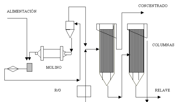
Figura N.º 12. Celdas-columna en todo el circuito de flotación
