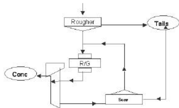
Figura N.º 11. Circuito convencional con celda-columna
