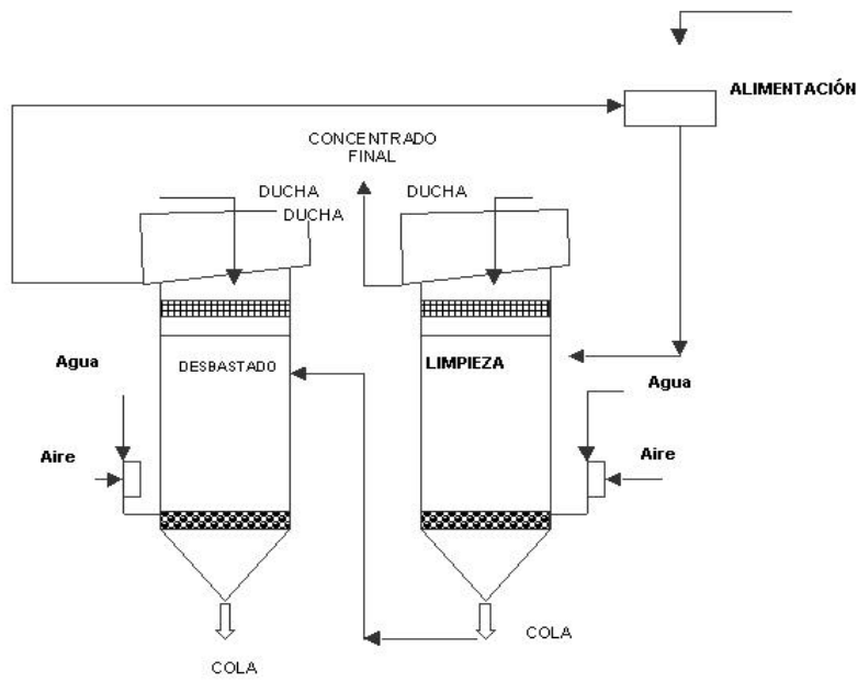
Figura N.º 6. Instalación en serie (18)
