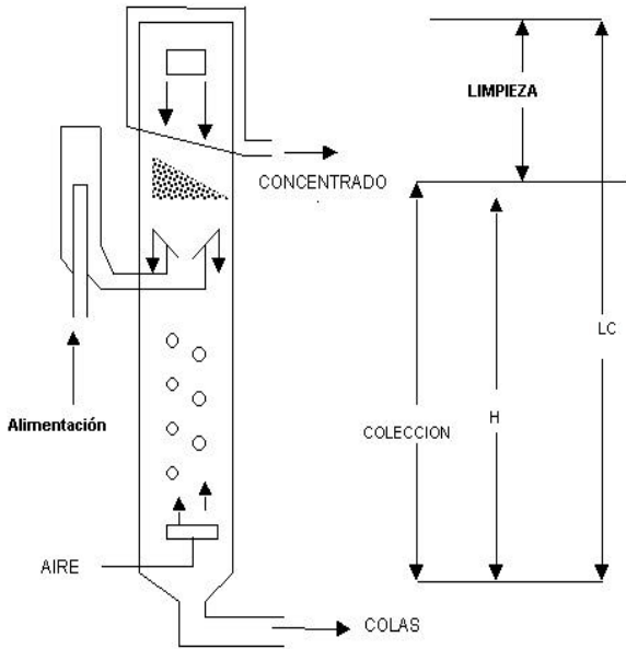
Figura N.º 1. Celda-columna (22)
