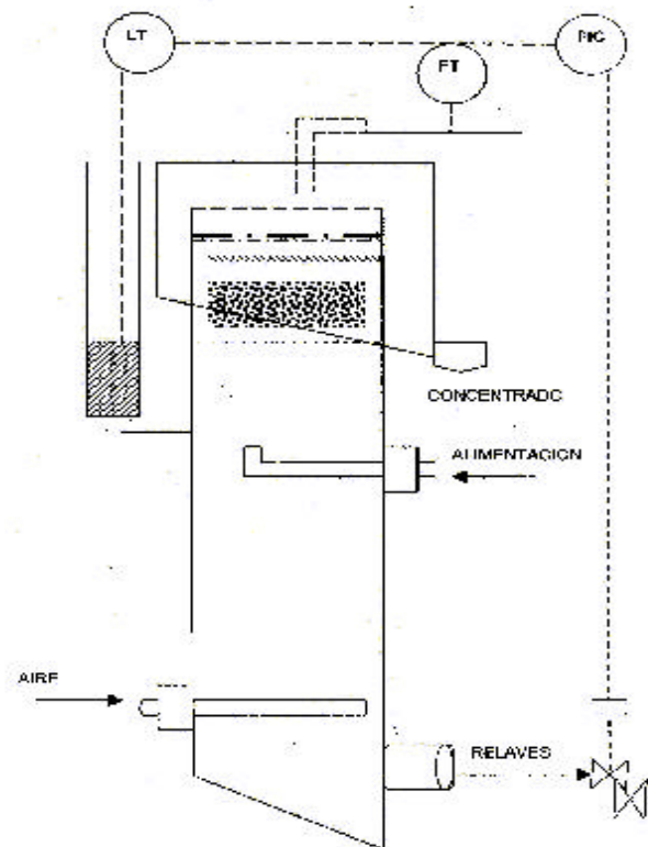
Figura N.º 5. Celda-columna con instrumentación básica (23)
