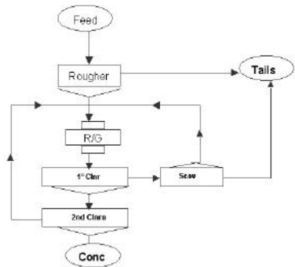
Figura N.º 10. Circuito convencional
