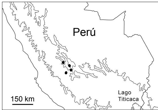
Figura 18.- Distribución geográfica de Hadruroides bustamantei n.sp. en el Perú. Cota de altitud 3000 m aproximadamente.
