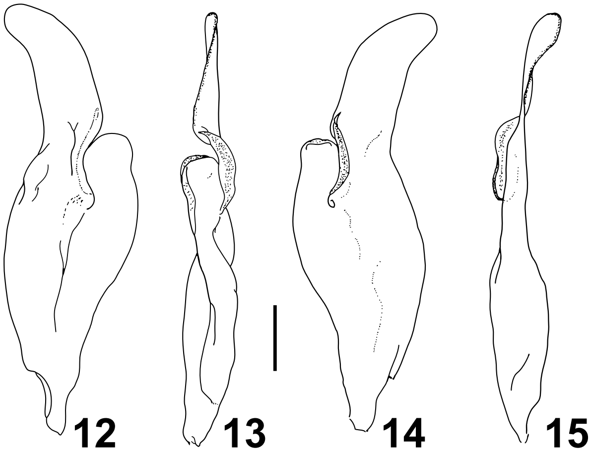
Figuras 12—15. - Hadruroides bustamantei n. sp., holotipo macho (MHNC): hemispermatóforo izquierdo; 12 , vista interna, 13 , vista frontal, 14 , vista externa, 15 , vista adfrontal. Escala: 1/2 mm.
