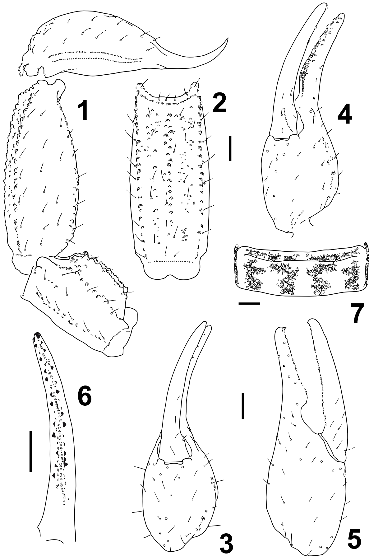
Figuras 1—7. - Hadruroides bustamantei n. sp.: 1—4, holotipo macho (MHNC); 1, segmento caudales IV—V y telson, vista lateral; 2, segmento caudal V, vista ventral; 3—5, pinza derecha, 3, vista ventral, 4, vista ventromedial, 5, vista lateral; 6, dedo móvil, detalle de la dentición. 7, paratipo hembra (MHNC): pigmento del tergito V. Escalas: 1 mm.
