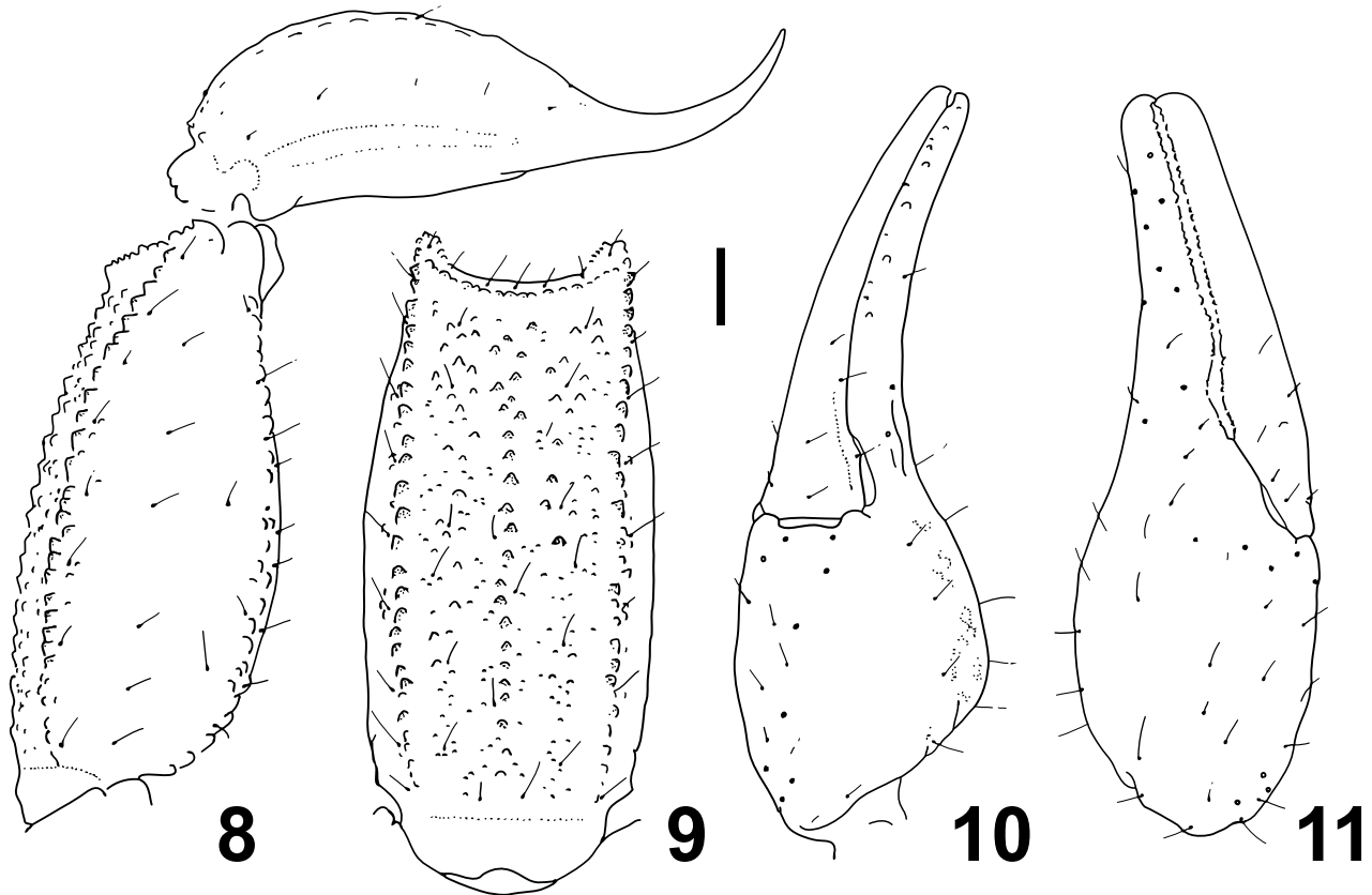
Figuras 8—11. - Hadruroides bustamantei n. sp., paratipo hembra (MHNC): 8 , segmento caudal V y telson, vista lateral; 9 , segmento caudal V, vista ventral; 10—11 , pinza derecha; 10 , vista ventromedial, 11 , vista lateral. Escala: 1 mm.
