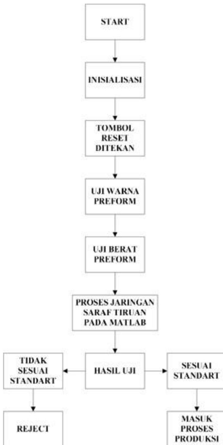
Gambar 2. Blok diagram cara kerja detektor standart preformbotol minuman
