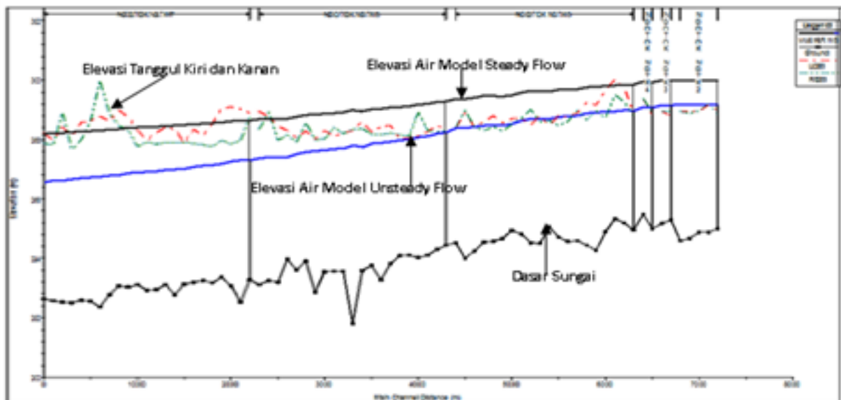
Gambar 9. Perbandingan Hasil Model aliran Steady Flow dan Unsteady Flow
