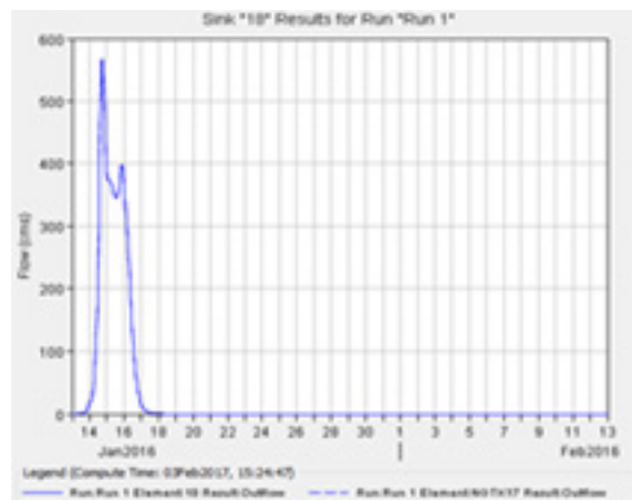
Gambar 6. Hidrograf Banjir Rencana
