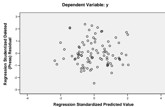
Gambar. 2. Uji Heterokedastisitas
