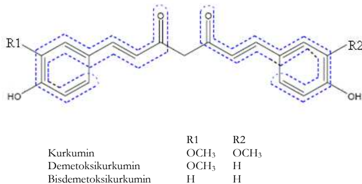
Gambar 1. Struktur kurkuminoid.
