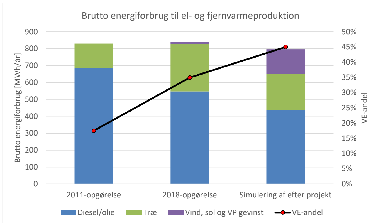
Figur 7 – Brutto energiforbrug i de to historiske opgørelser og det simulerede fremtidige scenarie
