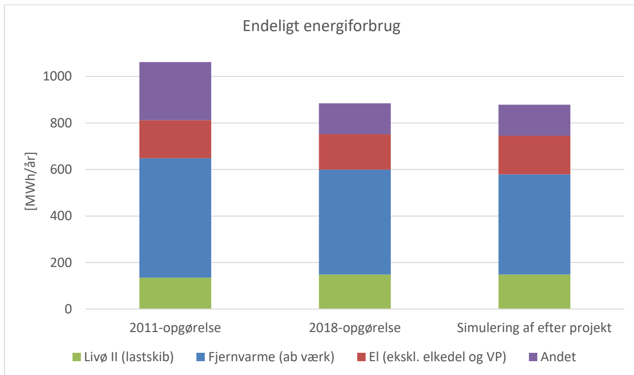
Figur 4 – Endelige energiforbrug på Livø i de to historiske opgørelser og det simulerede fremtidige scenarie
