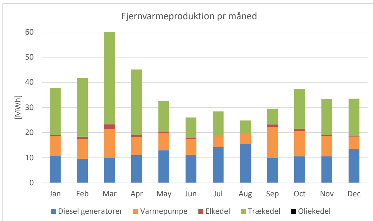
Figur 6 – Simuleret månedlig fjernvarmeproduktion
