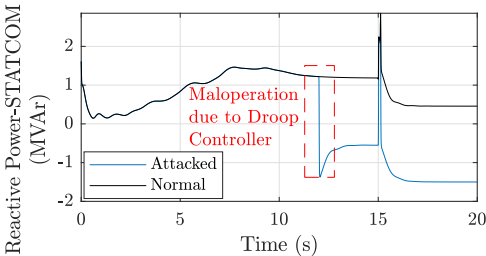
(d) Reactive Power from STATCOM.
