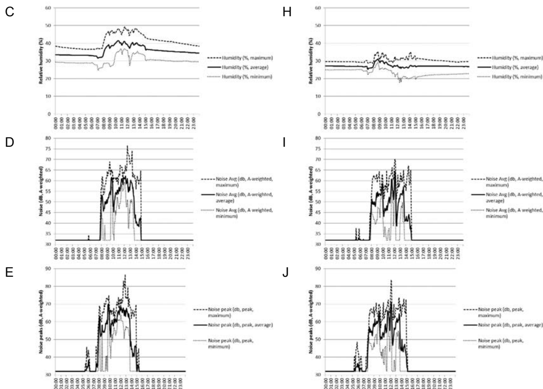
Figur 7: Maksimum, gennemsnit og minimumsværdier som indeklimaparametrene CO 2 (A og F), temperatur (B og G), fugtighed (C og H) og støj (D, E, I og J) i lokale 12 hv. uge 48, d. 28. november til 4. december 2017 (A-F) og uge 12, d. 20. til 26. marts 2017 (G-J). Data medtaget i figurerne er beregnet for dagene mandag til fredag (hverdagene).
