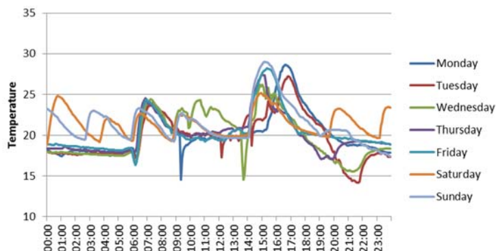
Figur 5. Figuren viser målingerne af temperaturen og dennes udsving i lokale 11 for dagene i uge 12. Henholdsvis mandag og onsdag ses kortvarigt temperatur fald til omkring 14.5°C, hvilket i evalueringen straffes hårdt og afspejles i den samlede evalueringsscore.
