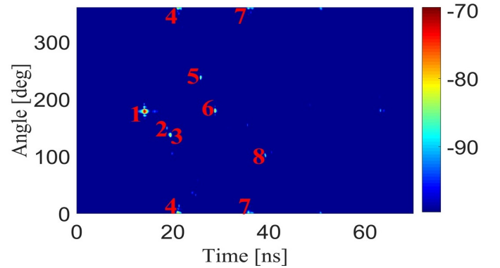
Fig. 4: PADP for the LOS scenario. Color bar units in dB.
