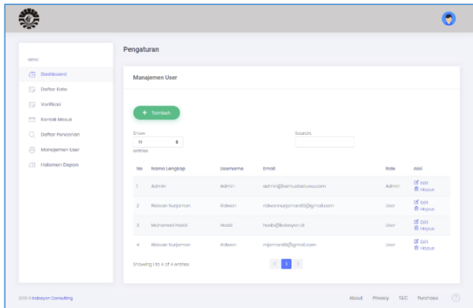
Gambar 23 Manajemen User
