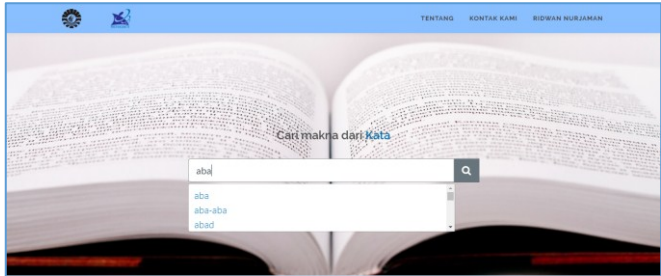
Gambar 11 Halaman Pencarian
