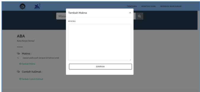
Gambar 13 Tambah Makna
