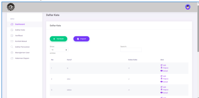
Gambar 17 Daftar Kata
