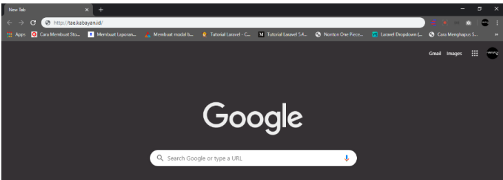
Gambar 1 Melakukan Akses
