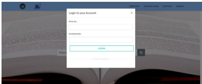
Gambar 6 Login
