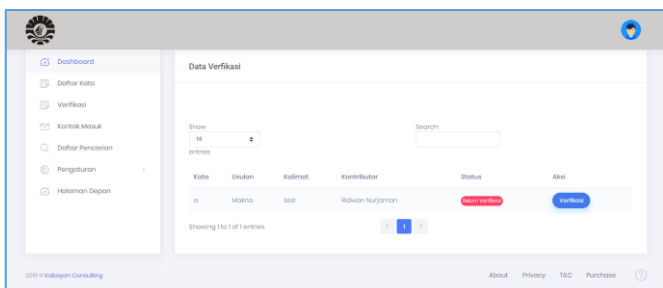
Gambar 20 Verfikasi
