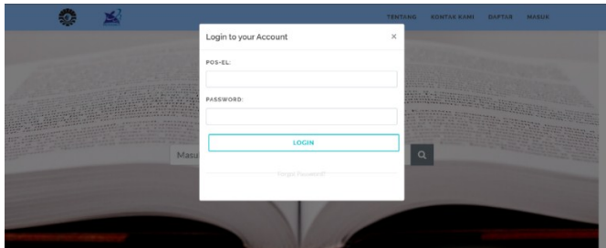
Gambar 15 Halaman Login
