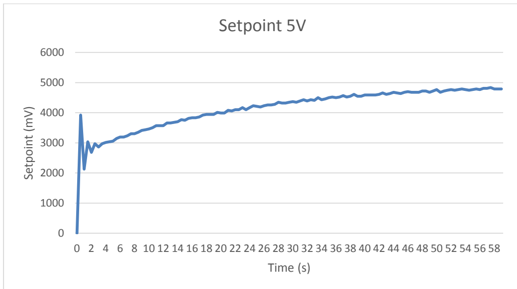
Gambar 3.5. Respon kontrol PID dengan setpoint 5 V
