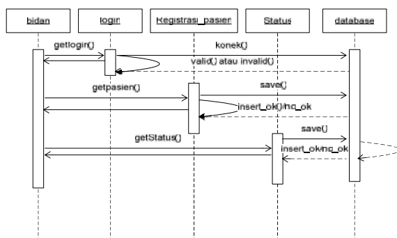
Gambar 8. Diagram Sequence data balita dan pemeriksaannya
