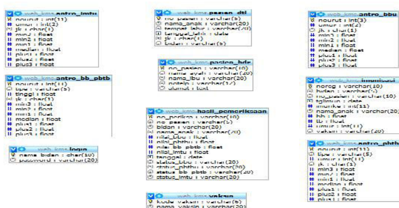
Gambar 10. Rancangan tabel-tabel pengolahan data KMS
