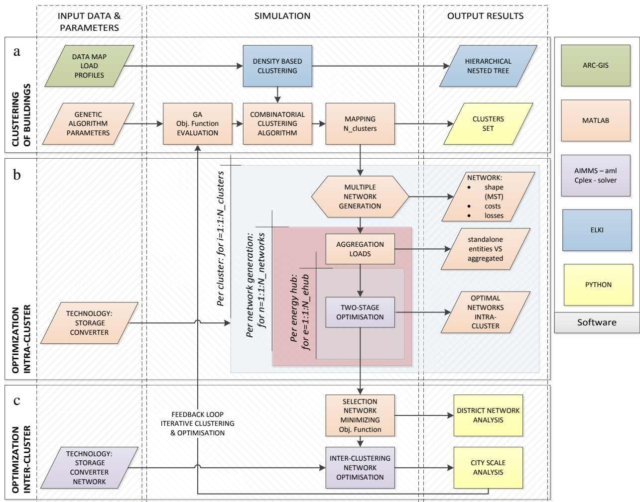
Fig. 2. Iterative multi-scale optimisation of DES
