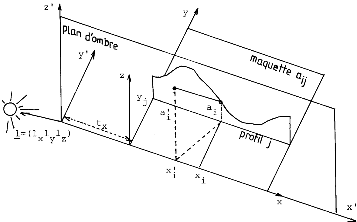
Fig.2.11 Projection d'un profil d'altitude a_i du système (x, y, z) dans le plan d'ombre du système (x', y', z')
