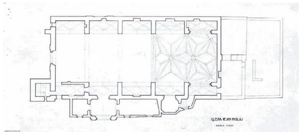
Planimetría del edificio levantada por Francisco Prieto- Moreno en 1937 [aipcf p 5872- 5873]
