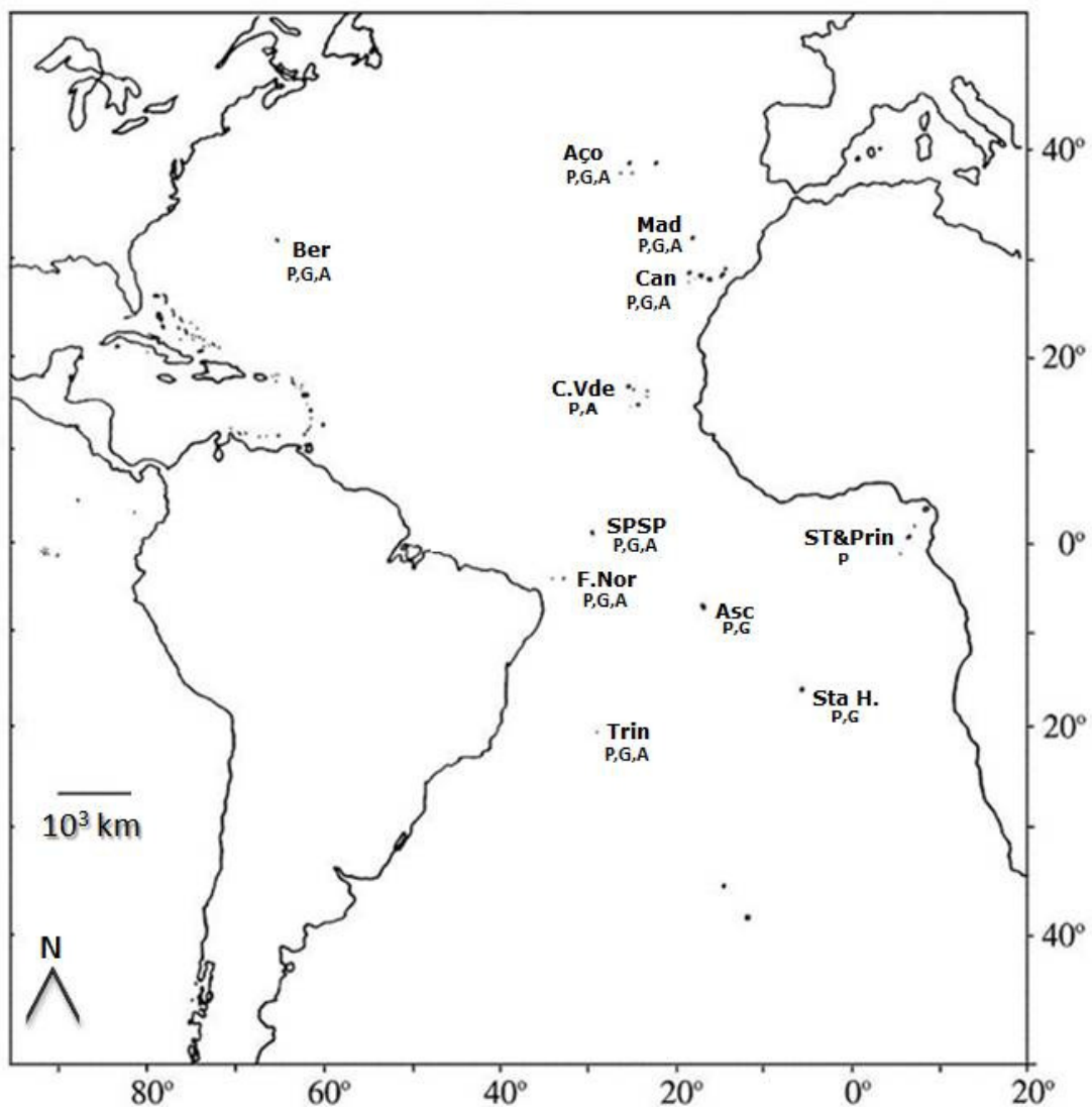
Figura 5. Ilhas do Oceânico Atlântico compreendidas no estudo e respectivos grupos marinhos estudados, sendo eles peixes recifais (P), gastrópodes (G) e macroalgas (A). Zona intertropical: Santa Helena (Sta H.); Ascensão (Asc); São Pedro e São Paulo (SPSP); Cabo Verde (C.Vde); Trindade (Trin); Cadeia de Montanhas de Fernando de Noronha (F.Nor); São Tomé e São Príncipe (ST&Prin). Zona temperada do norte: Bermudas (Ber); Canárias (Can); Açores (Aço); Madeira (Mad).
