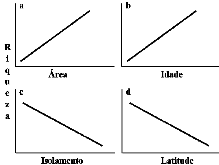
Figura 2. Padrões biogeográficos de distribuição de riqueza de espécies apontados pela literatura. a. Relação positiva riqueza-área; b. Relação positiva riqueza-idade; c. Relação negativa riqueza-isolamento; d. Relação negativa riqueza-latitude.
