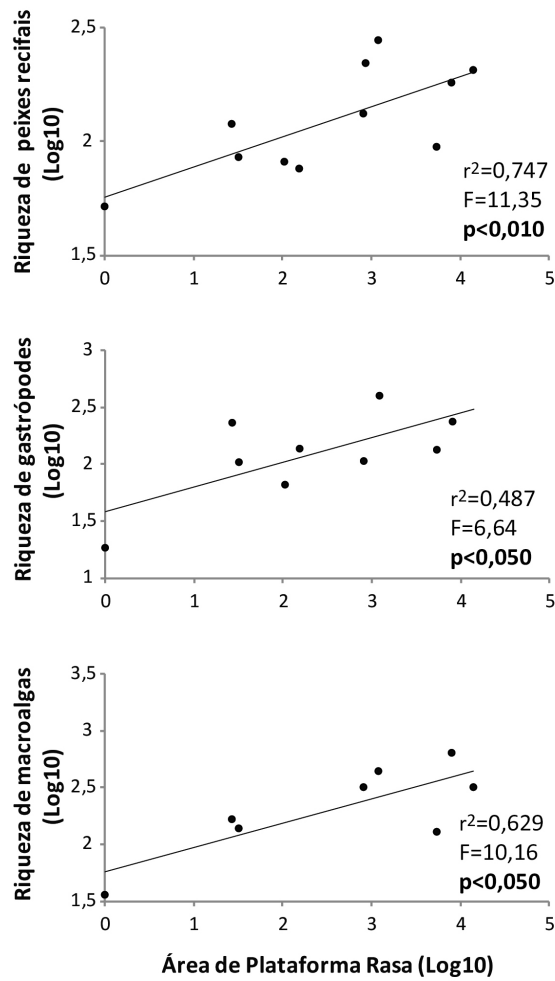
Figura 9. Relação entre riqueza de espécies e área de plataforma rasa para os três grupos marinhos: peixes recifais, gastrópodes e macroalgas.
