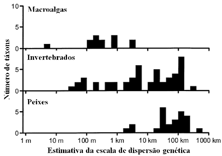
Figura 4. Dispersão de propágulos de macroalgas, invertebrados e peixes marinhos (Kinlan & Gaines, 2003).
