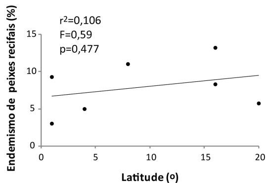
Figura 10. Relação entre porcentagem de endemismo de peixes recifais e latitude.
