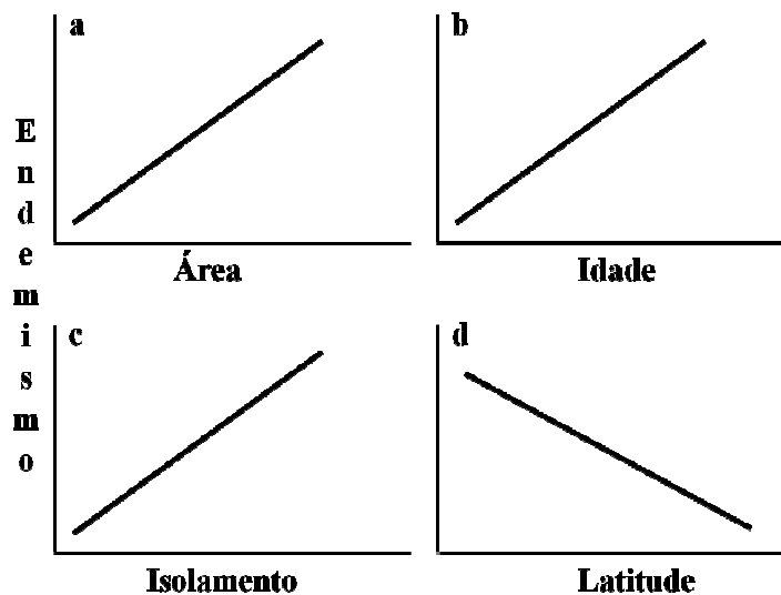
Figura 3. Padrões biogeográficos de distribuição de endemismo apontados pela literatura. a. Relação positiva endemismo-área; b. Relação positiva endemismo-idade; c. Relação positiva endemismo-isolamento; d. Relação negativa endemismo-latitude.
