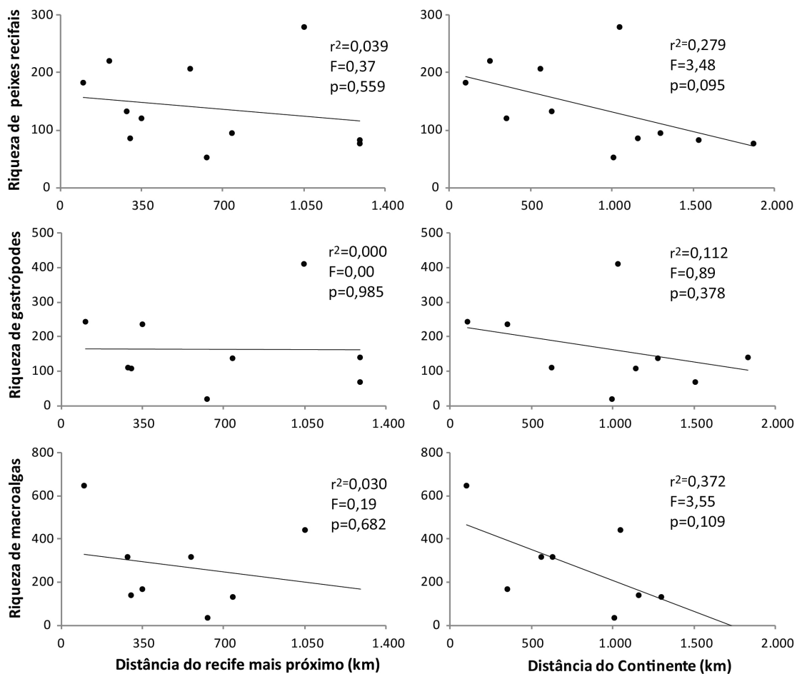
Figura 7. Relação entre riqueza de espécies e as distâncias do ambiente recifal mais próximo (à esquerda) ou do continente mais próximo (à direita) para grupos marinhos de peixes recifais, gastrópodes e macroalgas.
