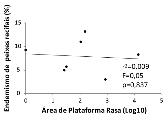
Figura 8. Relação entre porcentagem de endemismo de peixes recifais e área de plataforma rasa.
