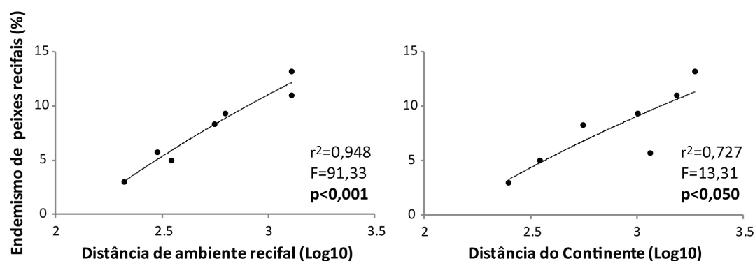
Figura 6. Relação entre a porcentagem de endemismo de peixes recifais e distâncias do ambiente recifal mais próximo (à esquerda) ou do continente mais próximo (à direita).
