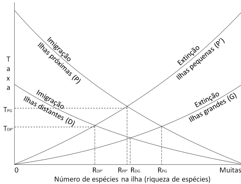
Figura 1. Modelo da Teoria de Biogeografia de Ilhas (MacArthur & Wilson, 1967). Taxa de imigração varia com o grau de isolamento da ilha e a taxa de extinção varia com o tamanho da ilha. Taxas semelhantes de imigração e extinção estabelecem uma riqueza de espécie (R) para a ilha, na qual ocorre o Turnover (T), caracterizado pela mudança na constituição de espécies da mesma.
