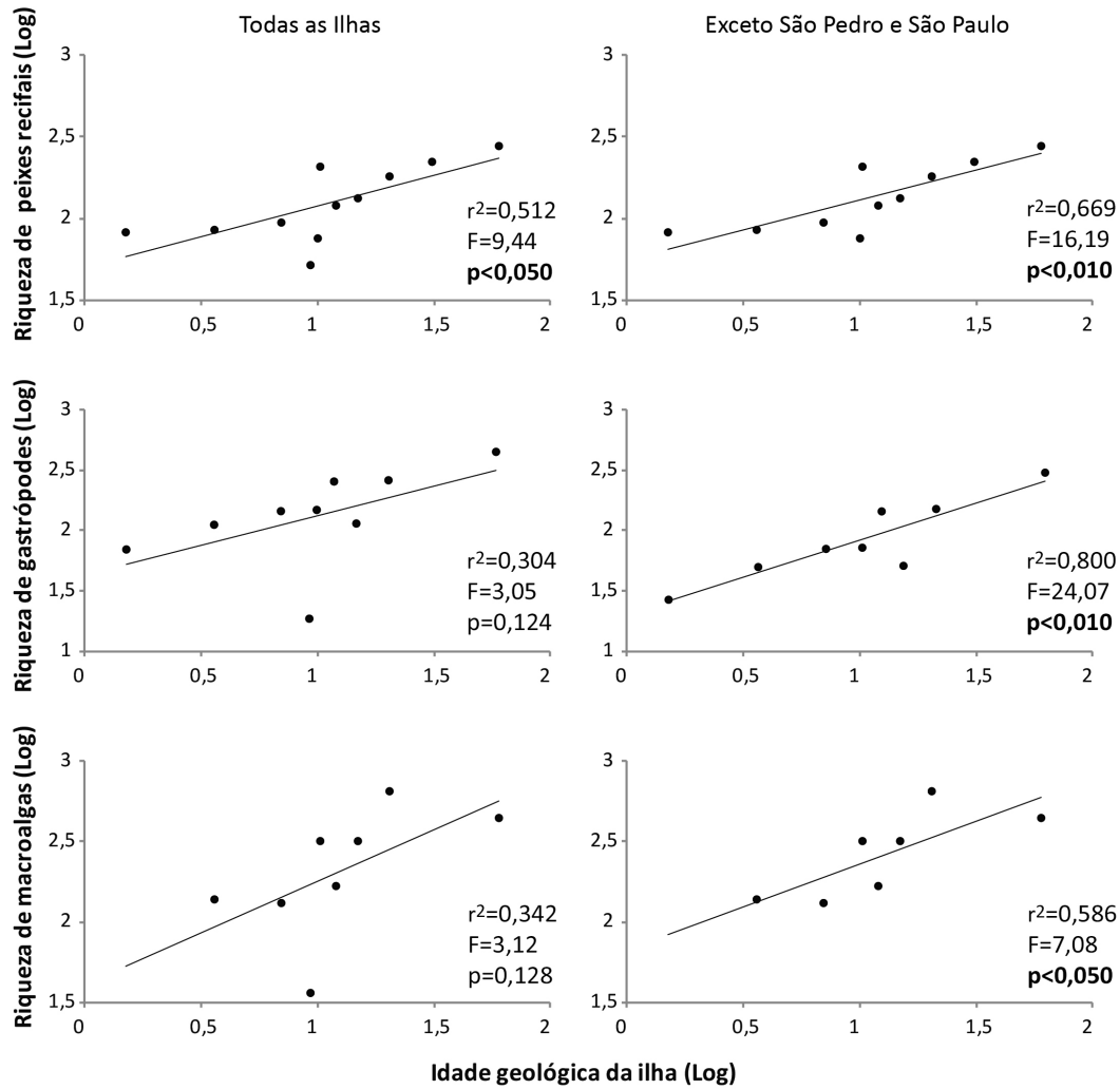
Figura 13. Relação entre riqueza de espécies e idade geológica das ilhas para peixes recifais, gastrópodes e macroalgas. Análises realizadas com dados de todas as ilhas (à esquerda) e excetuando outliers - ilha São Pedro e São Paulo (à direita).
