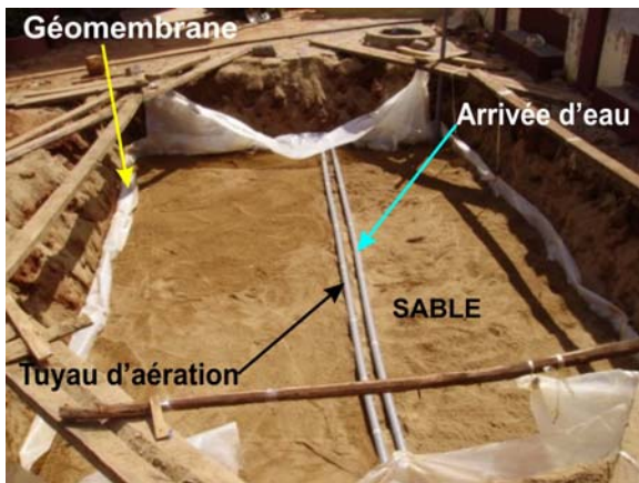
Remplissage du REEPS fini
