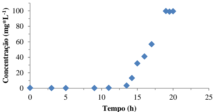
Figura 32 - Curva de adsorção do azul de metileno na areia em coluna de leito fixo: concentração de corante por espectroscopia de UV-Visível de acordo com o tempo.
