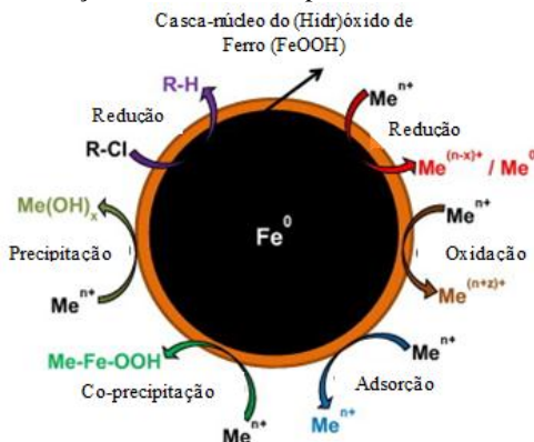
Figura 2- Estrutura casca-núcleo de nZVI descrevendo vários mecanismos para a remoção de metais e compostos clorados
