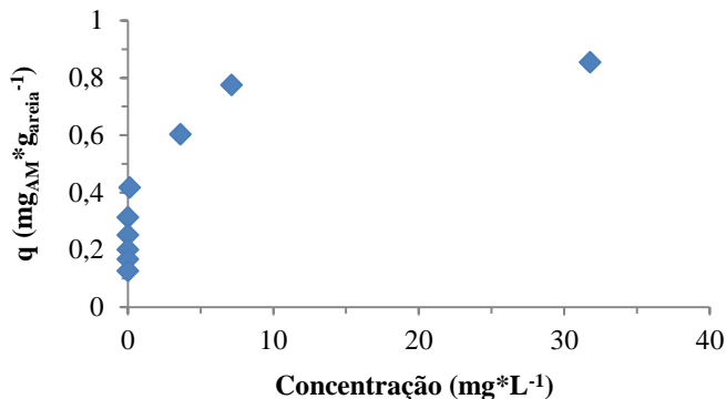
Figura 28 - Curva de adsorção do azul de metileno na areia: quantidades de corante adsorvido de acordo com a concentração de corante no equilíbrio.
