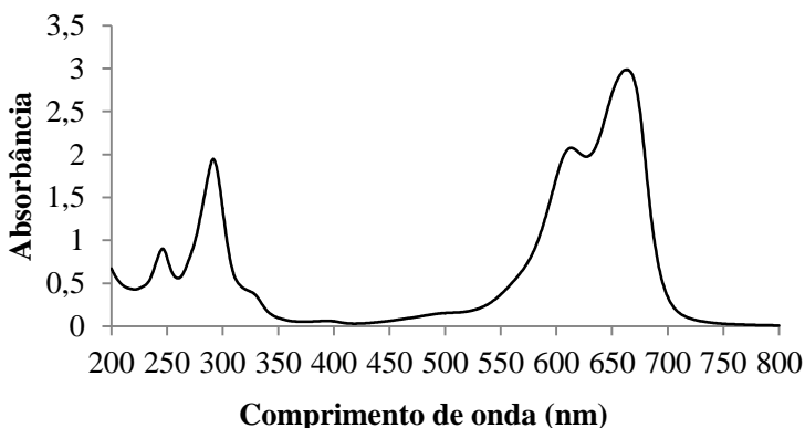
Figura 10- Espectro de absorbância do corante azul de metileno.
