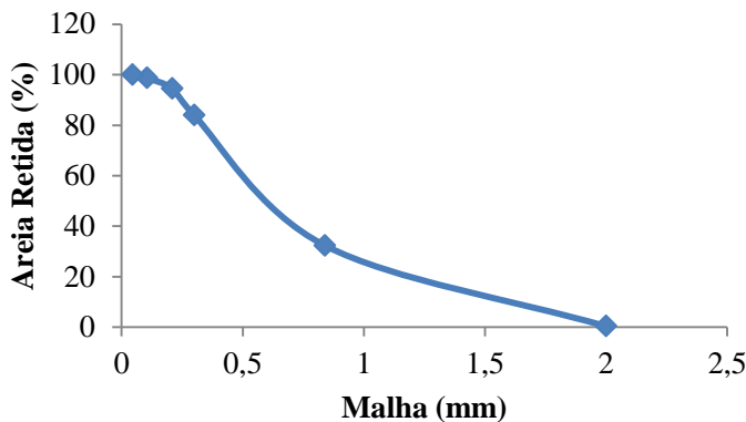
Figura 22 - Curva granulométrica da areia
