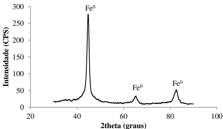
Figura 15 - Difratograma de raios-X das nZVI sintetizadas através da reação do \text{FeCl}_3 e \text{NaBH}_4
