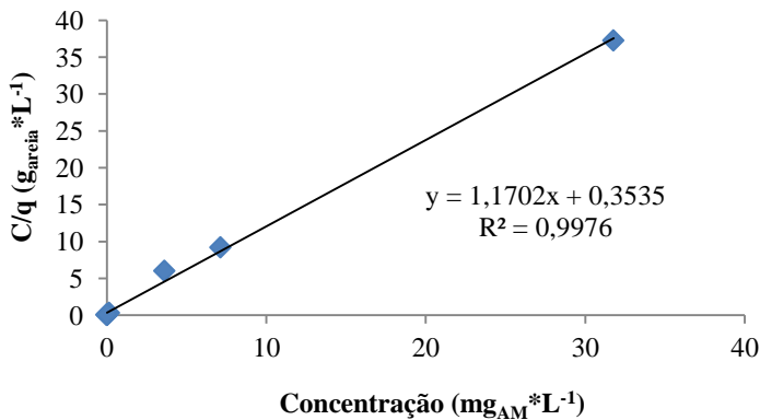
Figura 29 - Linearização dos dados experimentais, segundo modelo proposto por Langmuir.
