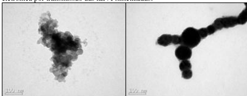
Figura 18 - Análise de estrutura e tamanho de partícula por microscopia eletrônica por transmissão das nZVI sintetizadas.
