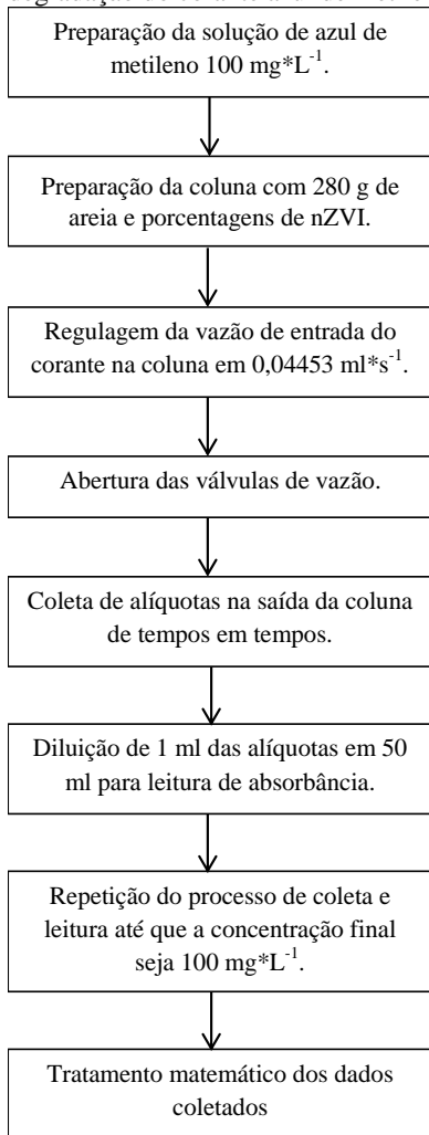
Figura 14- Fluxograma da metodologia adotada nos experimentos de degradação do corante azul de metileno pelas nZVI em coluna de leito fixo.
