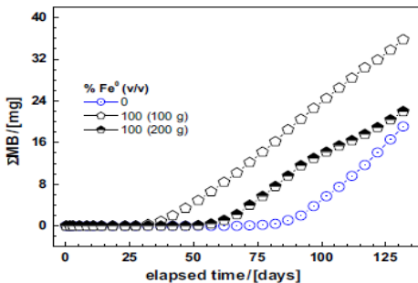
Figura 5 - Efeito do uso de \text{Fe}^0 sobre o desempenho da coluna de areia para descoloração do azul de metileno.
