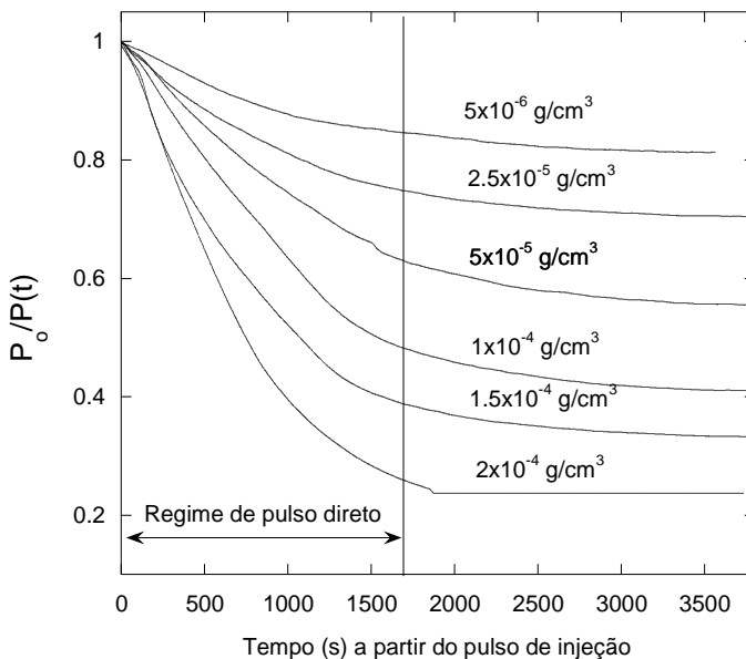
Figura 33 - P_0/P(t) para diferentes concentrações de esferas, Q = 0,8 \text{ cm}^3 \text{ min}^{-1} .
