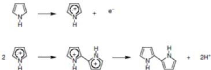
Figura 13 - Etapas da polimerização do Pirrol.
