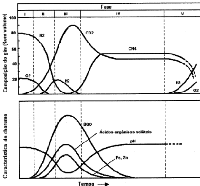
Figura 3.1 - Fases de formação do biogás de aterro Fonte: Tchobanoglous, Theisen & Vinil (1993)
